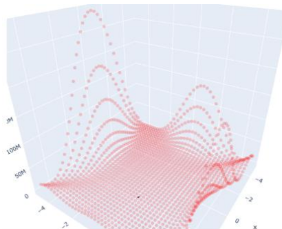
Figura11 Camino decreciente sobre la superficie de Goldstein-Price con 20.000 iteraciones
