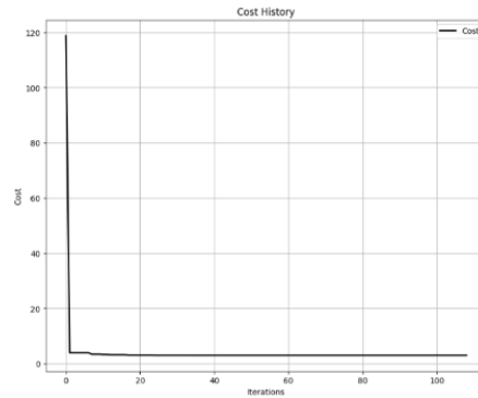
Figura21 Optimización de la función Goldstein con Optimización de Partículas
