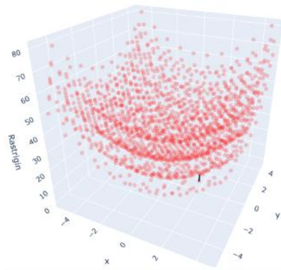
Figura8 Camino decreciente sobre la superficie de Rastrigin con 20.000 iteraciones
