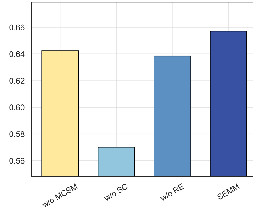
CPC
