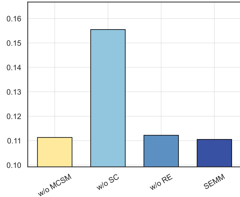
JSD
