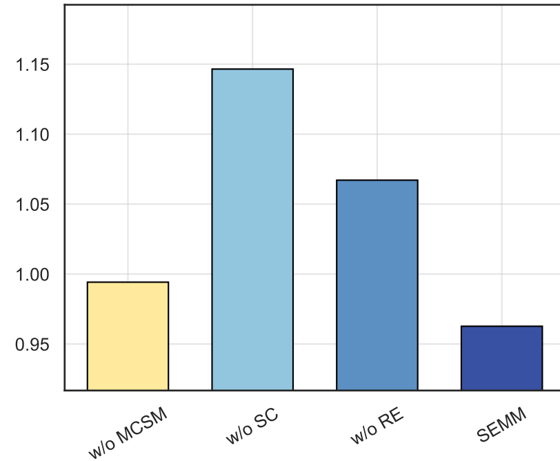
MAE
