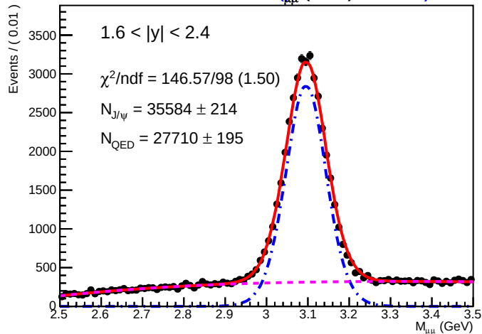
SA RooPlot of 7 M μμ (GeV).01635)
