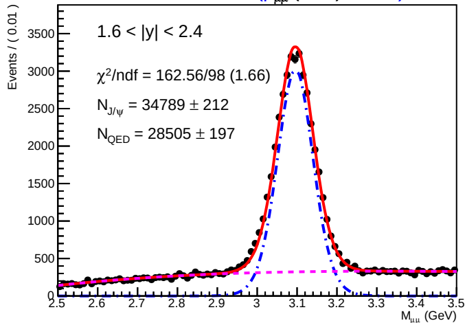
SA-RooPlot of M_{\mu\mu} (GeV) 01140)
