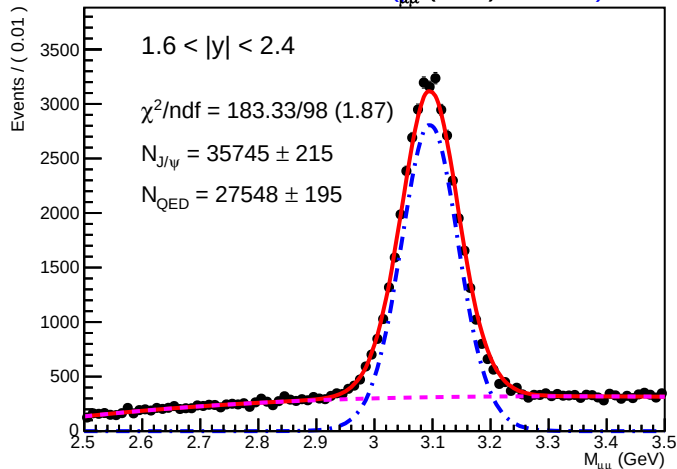
SA RooPlot 16 Mpa(GeV).01730)
