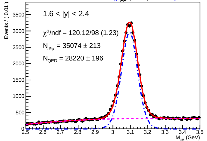
SA-RooPlot of M_{\mu\mu} (GeV) 01325)
