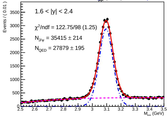
SA RooPlot of 7 M μμ (GeV).01535)
