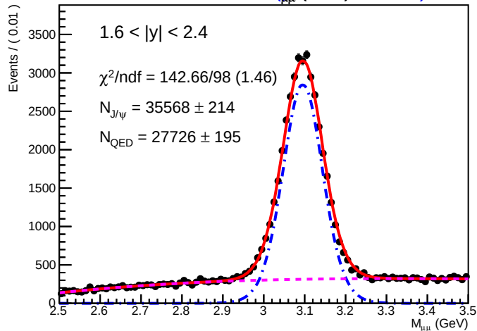
SA RooPlot of 5 M μμ (GeV).01625)
