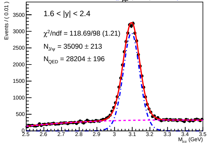
SA-RooPlot of M_{\mu\mu} (GeV) 01335)
