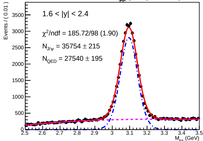
SA RooPlot 17 Mpa(GeV).01735)
