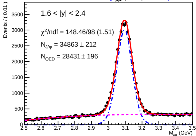
SA-RooPlot of M_{\mu\mu} (GeV) 01190)
