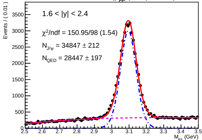
SA-RooPlot of M_{\mu\mu} (GeV) 01180)
