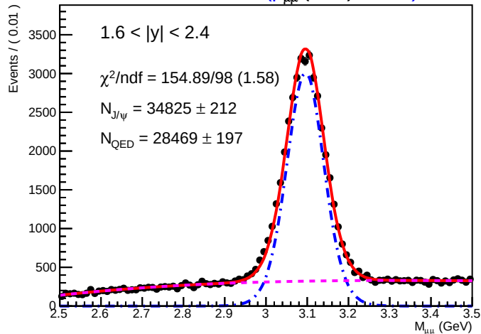
SA Root Plot of M_{\mu\mu} (GeV) 01165)
