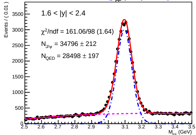
SA-RooPlot of M_{\mu\mu} (GeV) 01145)
