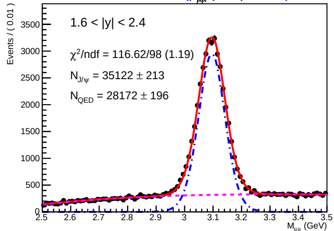
SA RooPlot of 'M μμ (GeV)' 01355)
