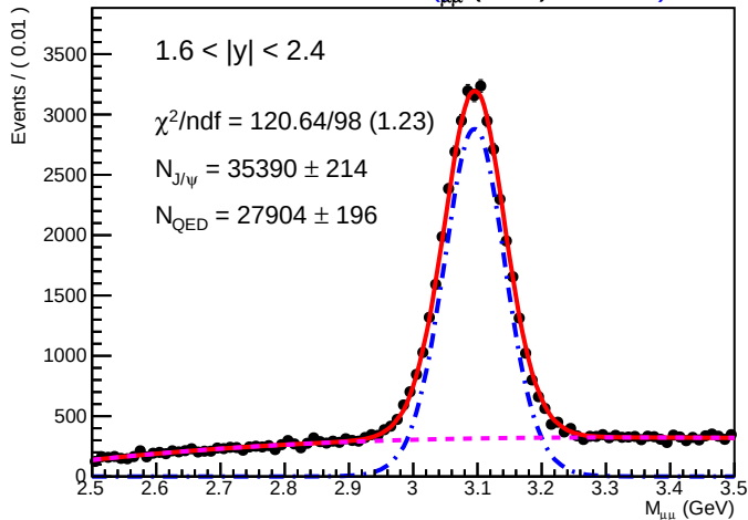
SA RooPlot of 4 M μμ (GeV).01520)
