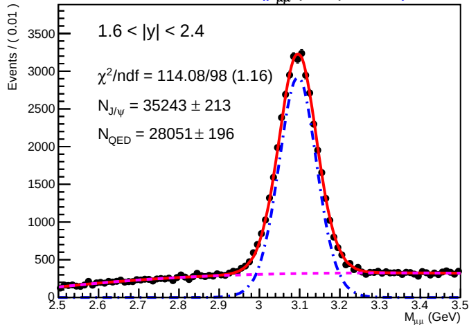
SA Root Plot of M_{\mu\mu} (GeV) 01430)
