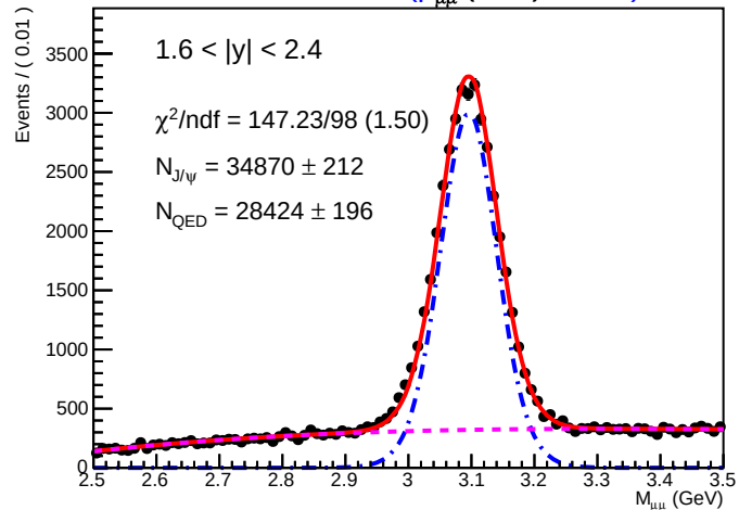
SA-RooPlot of M_{\mu\mu} (GeV) 01195)
