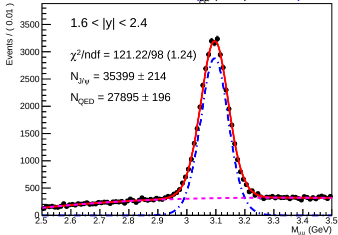
SA RooPlot of 5 M μμ (GeV).01525)
