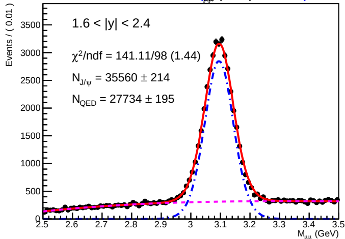
SA RooPlot of 4 M μμ (GeV).01620)
