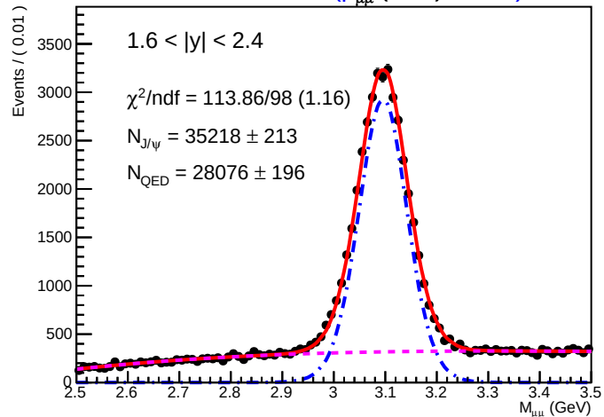
SA-RDPlot of M_{\mu\mu} (GeV) 01415
