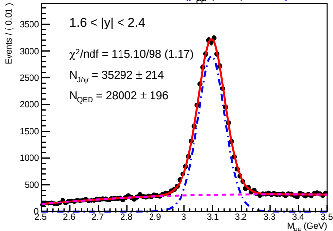
SA-RooPlot of M_{\mu\mu} (GeV) 01460)
