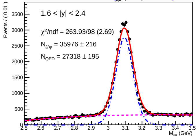
SA RooPlot of 3M μμ (GeV) (0.1865)
