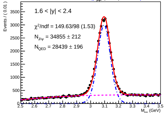
SA-RooPlot of M_{\mu\mu} (GeV) 01185)
