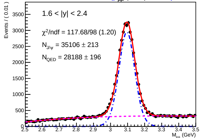
SA RooPlot of 'M μμ (GeV)' 01345)
