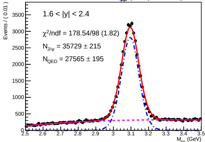
SA RooPlot 14 Mpa(GeV).01720)
