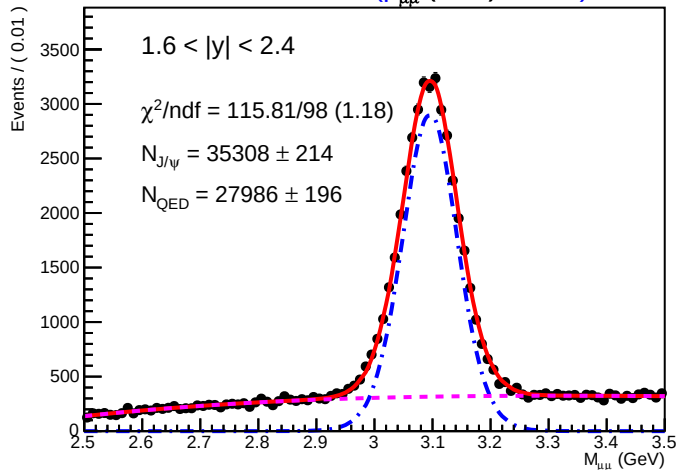
SA-RooPlot of M_{\mu\mu} (GeV) 01470)
