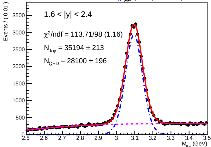
SA-RDPlot of M_{\mu\mu} (GeV) 01400
