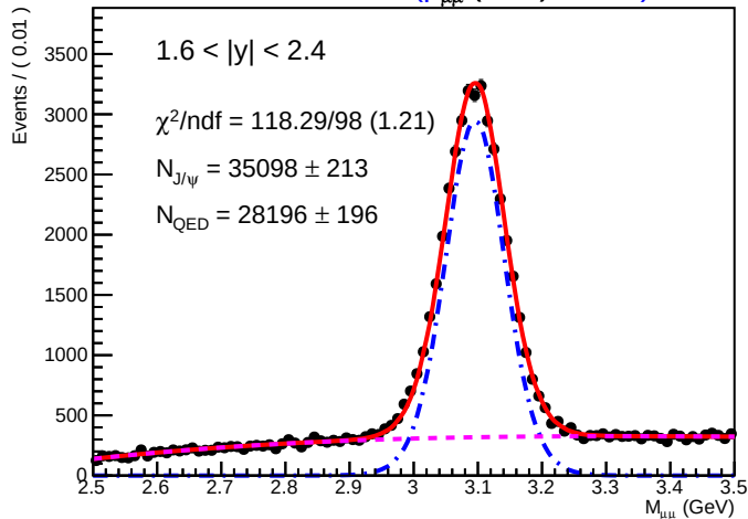
SA RooPlot of 'M μμ (GeV)' 01340)
