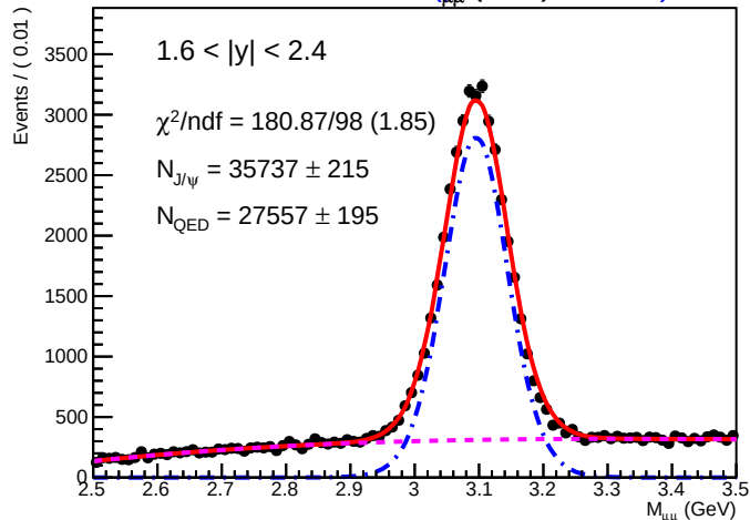
SA RooPlot 15 Mpa(GeV).01725)
