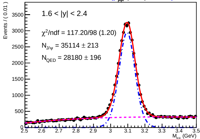
SA RooPlot of 'M μμ (GeV)' 01350)
