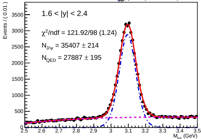
SA RooPlot of 6 M μμ (GeV).01530)
