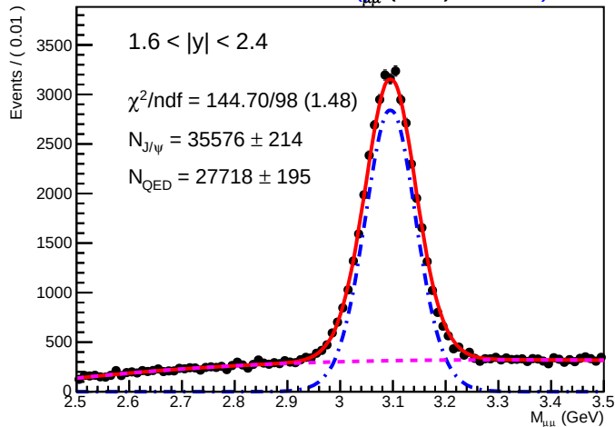
SA RooPlot of 6 M μμ (GeV).01630)
