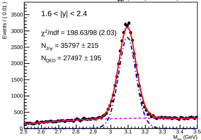
SA RooPlot of 2M μμ (GeV) 0.01760
