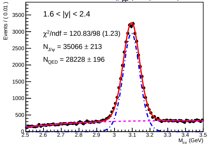
SA-RooPlot of M_{\mu\mu} (GeV) 01320)
