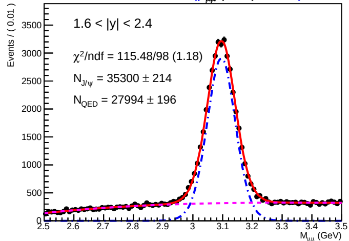
SA-RooPlot of M_{\mu\mu} (GeV) 01465)
