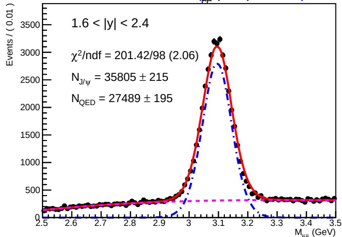
SA RooPlot of 3M μμ (GeV) 0.01765
