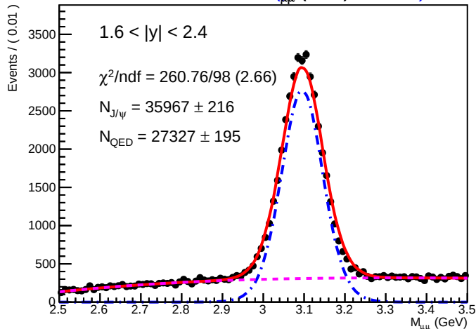
SA RooPlot of 2M μμ (GeV) (0.1860)
