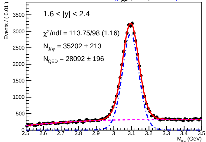
SA-RDPlot of M_{\mu\mu} (GeV) 01405
