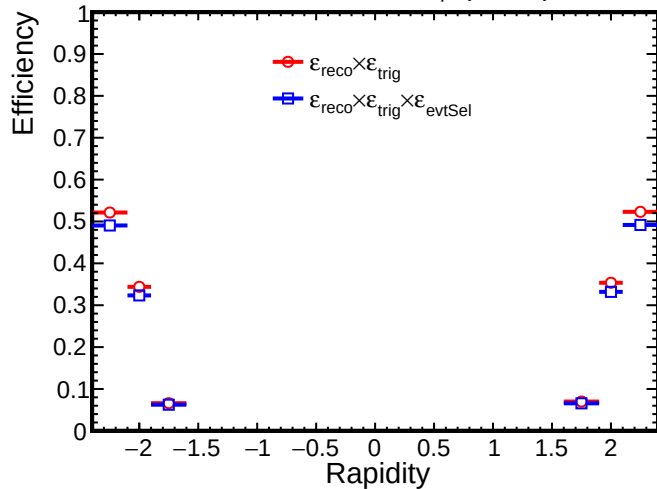
Coherent J/\psi (XnXn)
