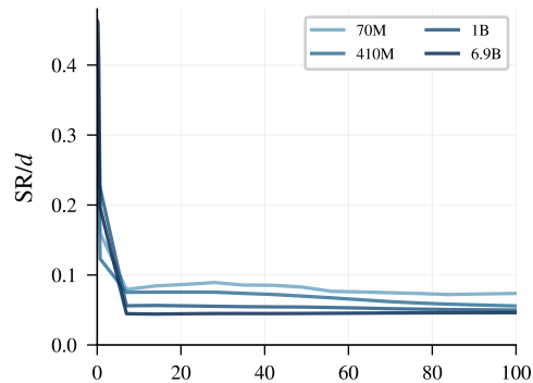
GPT-NeoX (Pythia)
