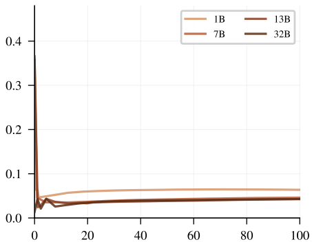
OLMo-2
