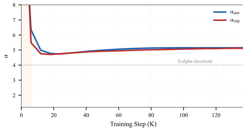
(d) Attn vs MLP decomposition — 6.9B
