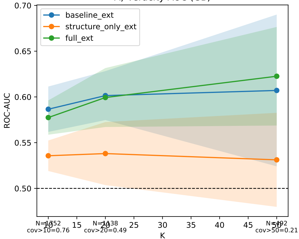
A) Veracity AUC (GB)
