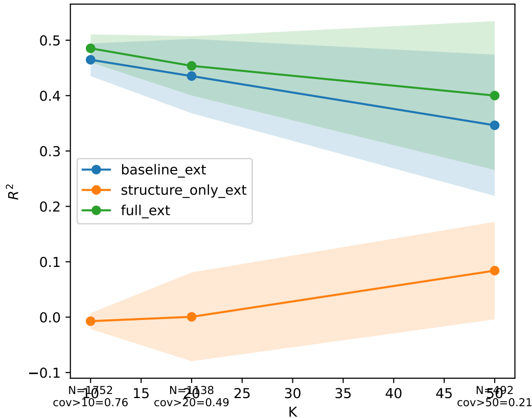
B) Reach R^2 (GBREG)
