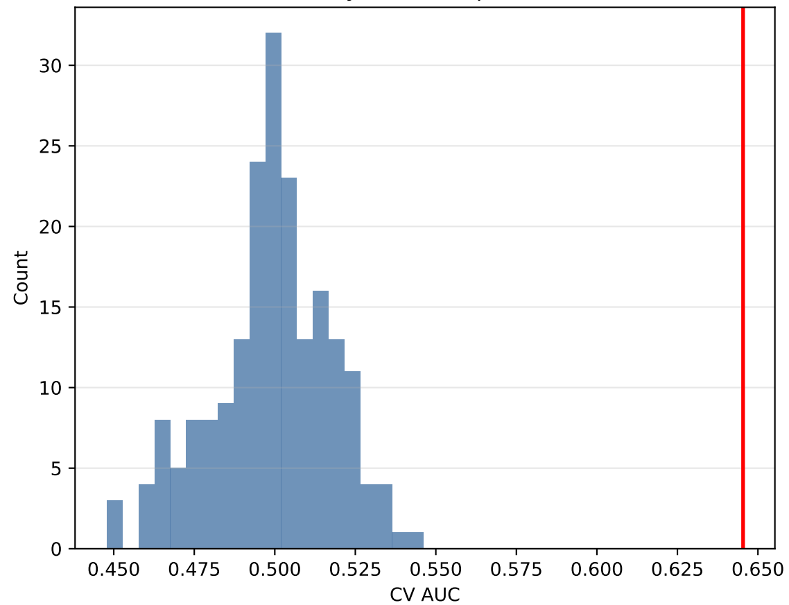
Veracity AUC null ( p=0.000 )
