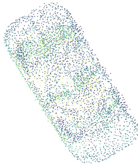
PU-GCN 4096
