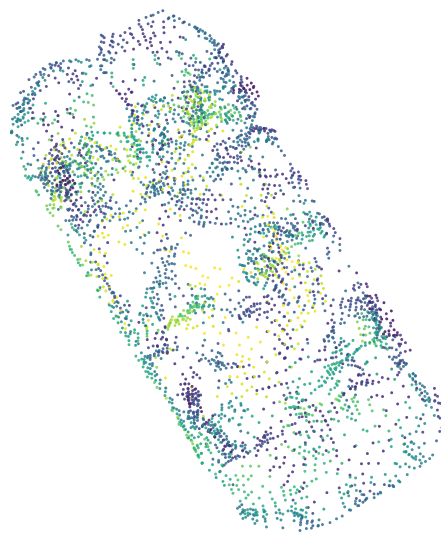
PDANS 4096
