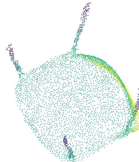
PU-GCN 4096
