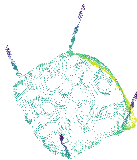
PDANS 4096
