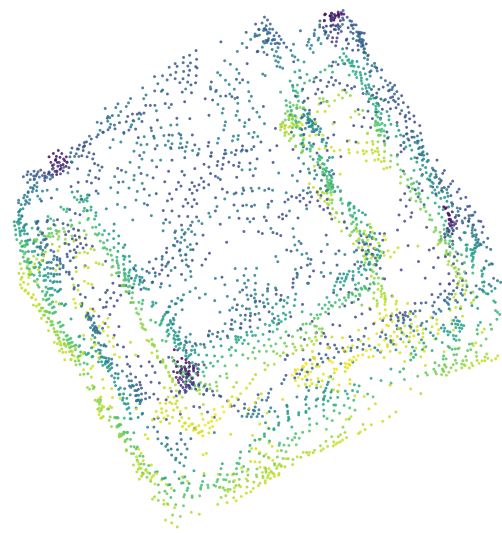
PDANS 4096
