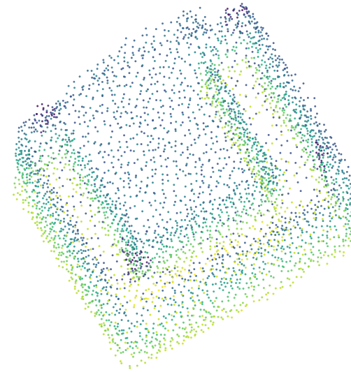
PU-GCN 4096
