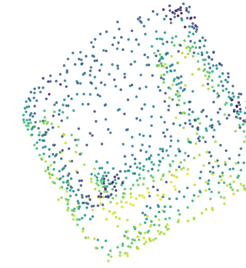
PU-GCN 1024
