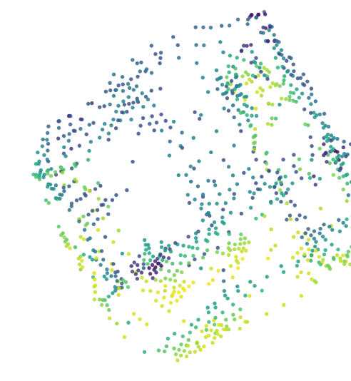
PDANS 1024
