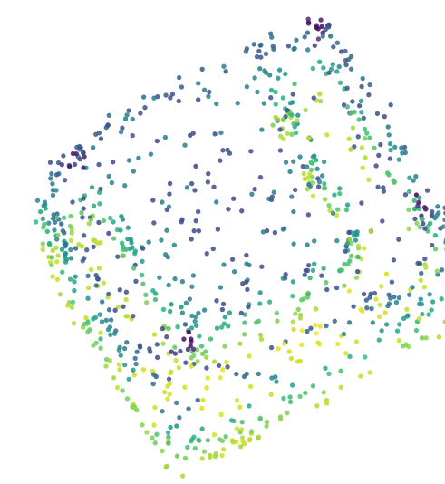
PU-Net 1024
