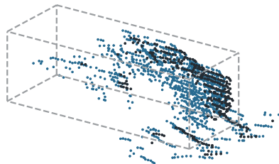
(d) PU-EF
