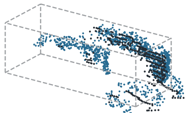
(d) PU-EF
