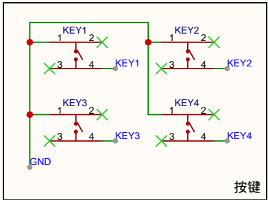
按键
