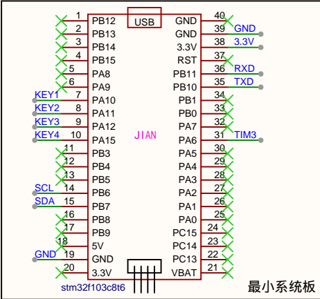
最小系统板
