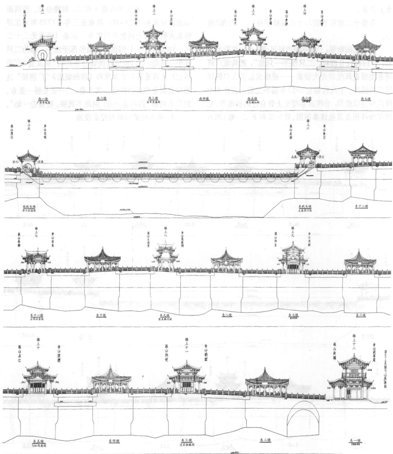
图5 广济桥亭台楼阁纵剖面图
