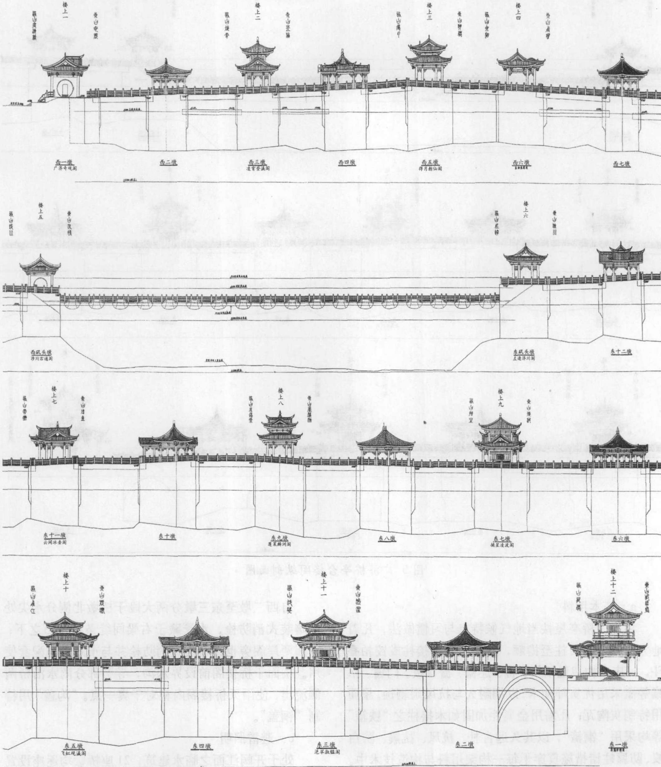
图4 广济桥亭台楼阁南立面图
