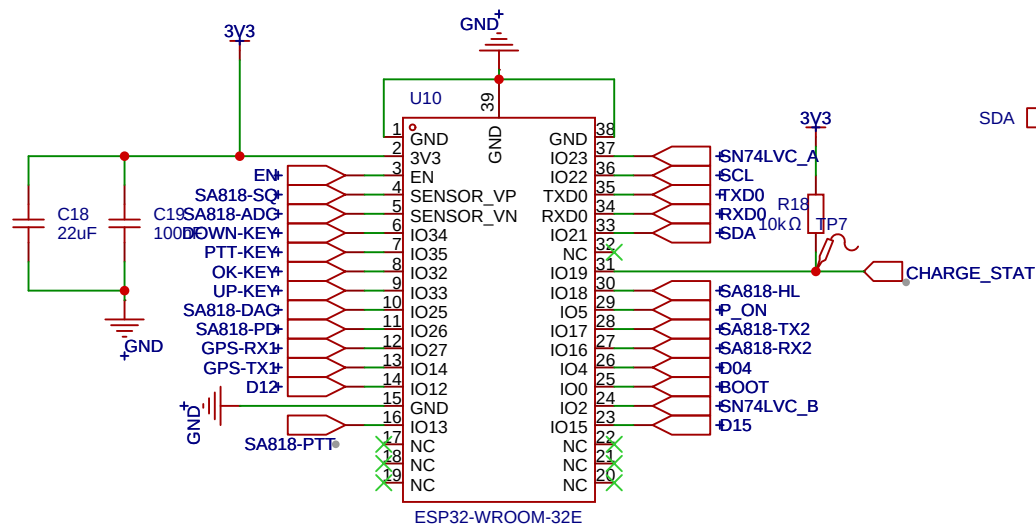
MCU
