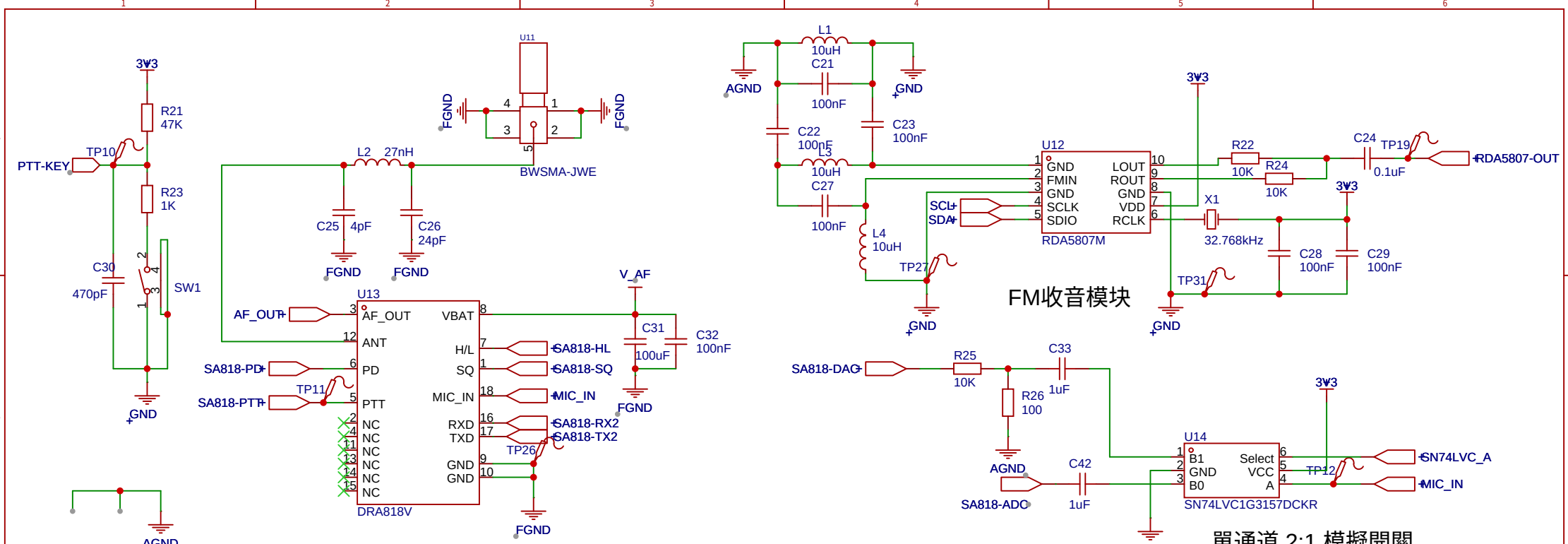
射频模块
