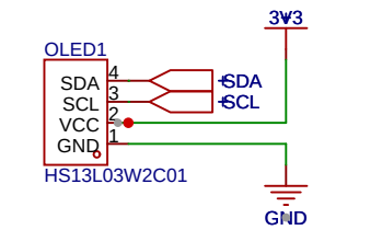
OLED接口
