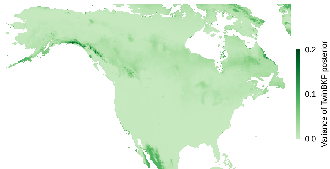
(d) TwinBKP – Prediction uncertainty
