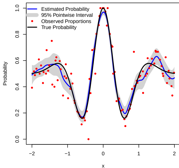
(d) BKP-ESS, n=100
