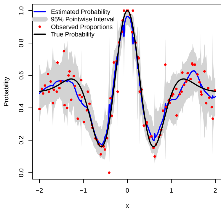
(f) LGP, n=100
