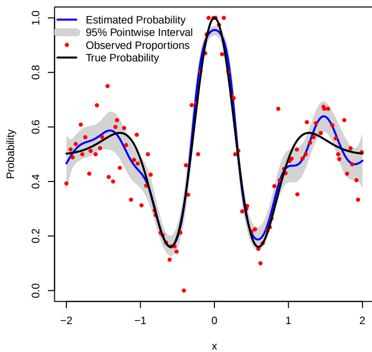
(f) LGP, n=100
