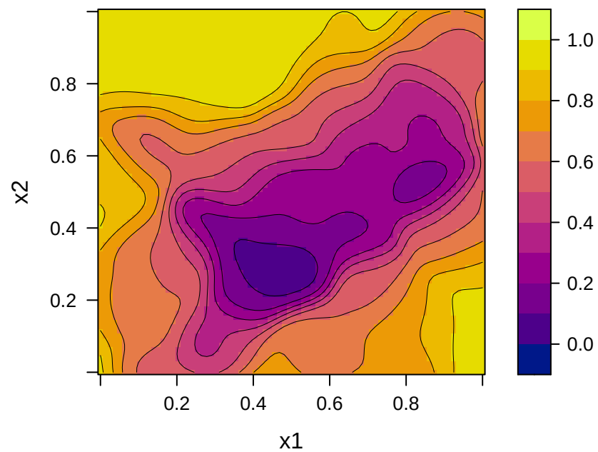
95% CI Lower
