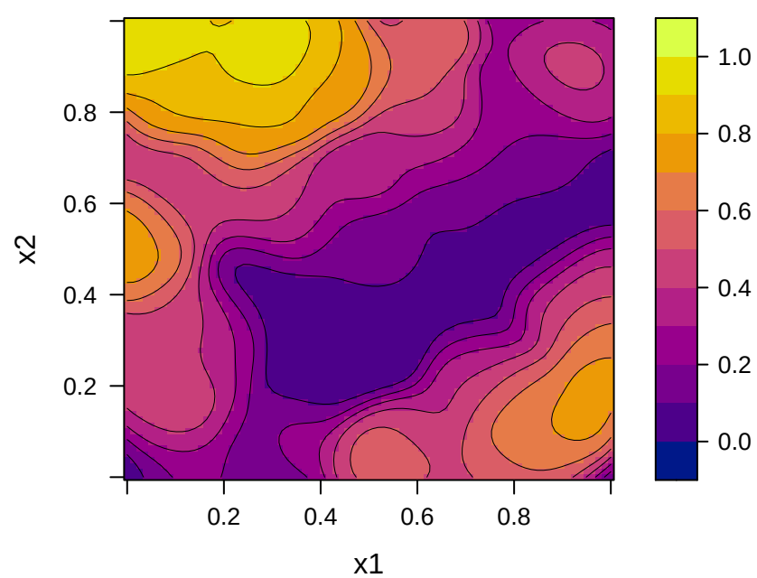
95% CI Lower
