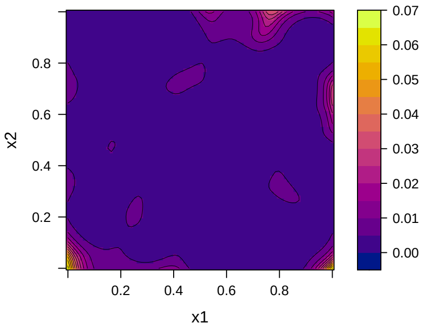
Posterior Variance
