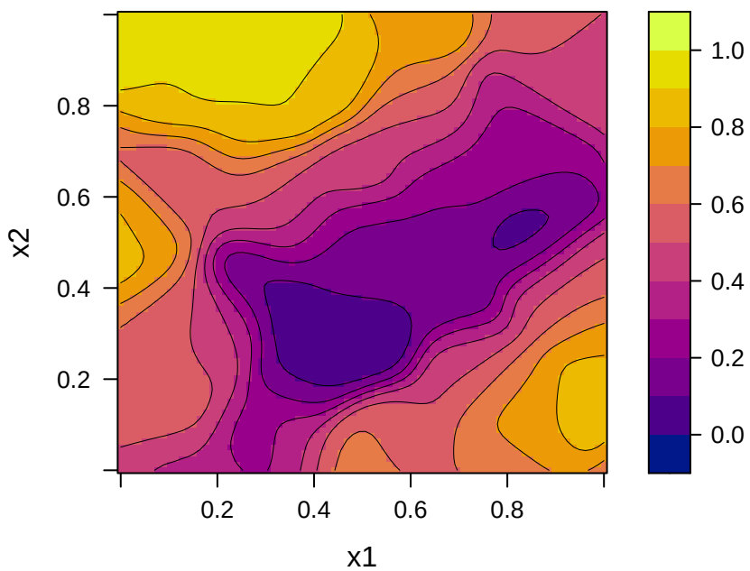
Posterior Variance
