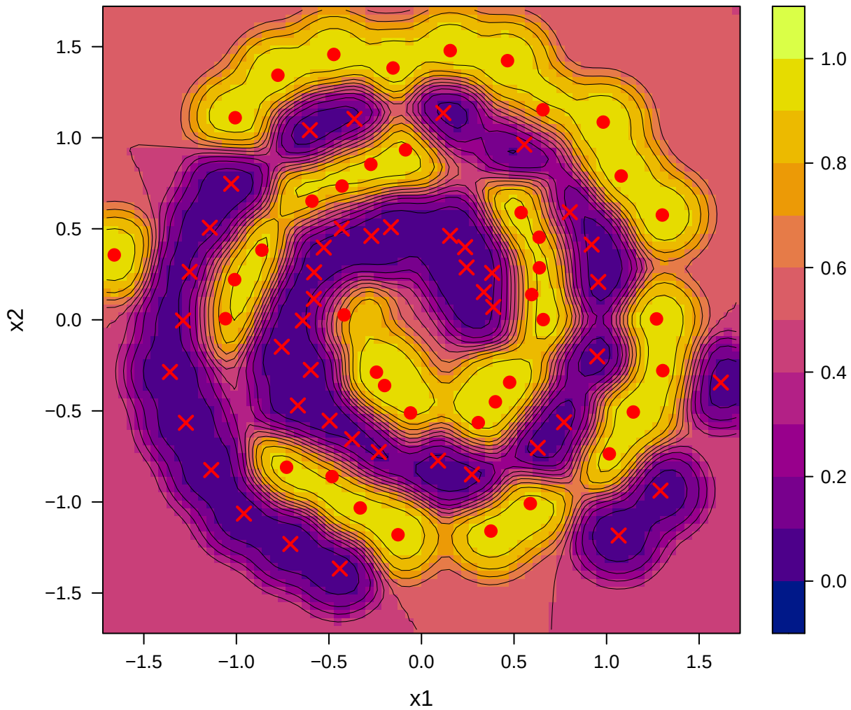
Posterior Mean
