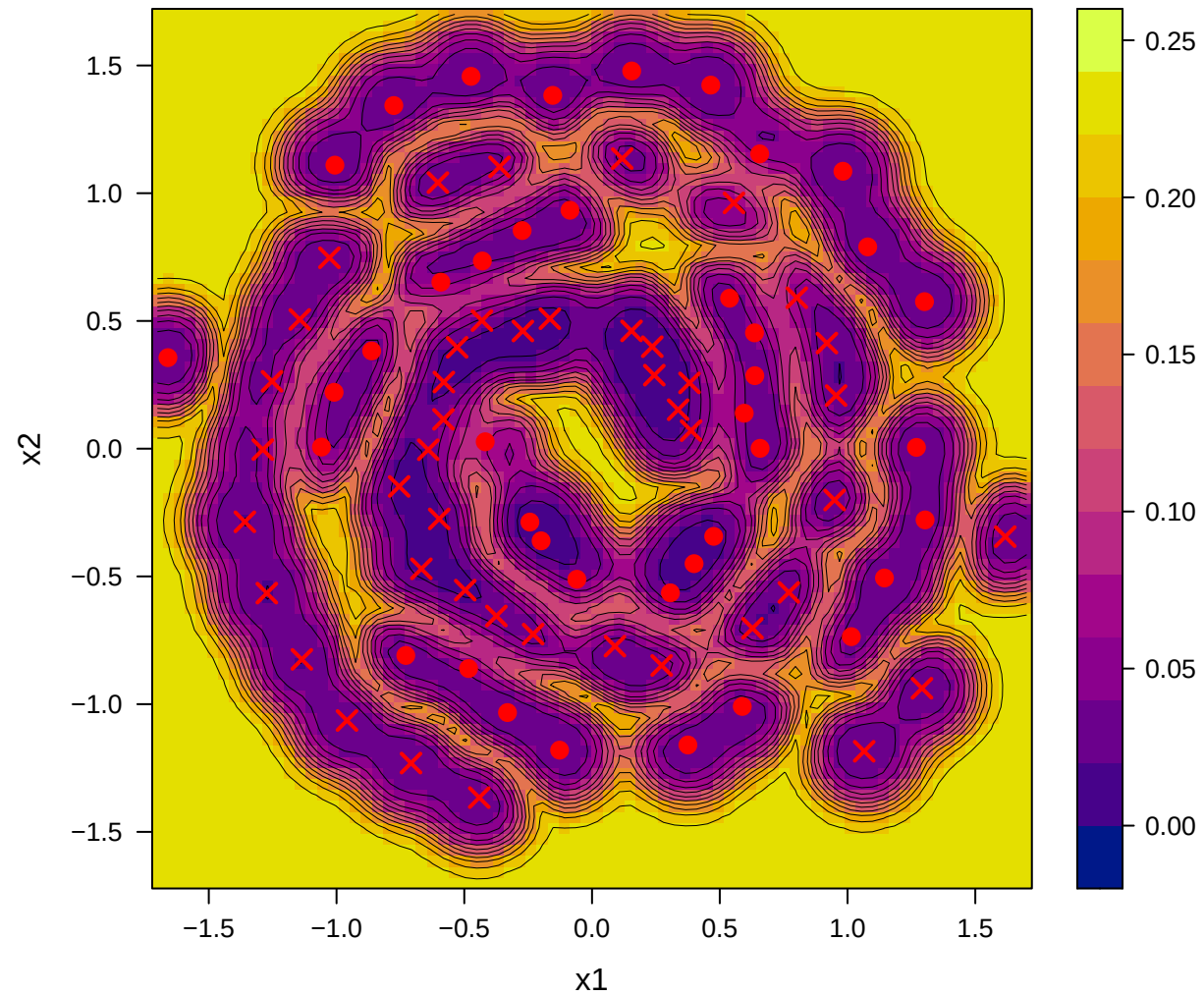
Posterior Variance
