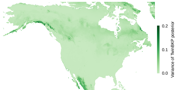
(d) TwinBKP – Prediction uncertainty
