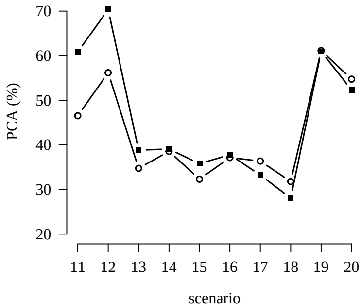
(d) PCA under \phi = 0.3
