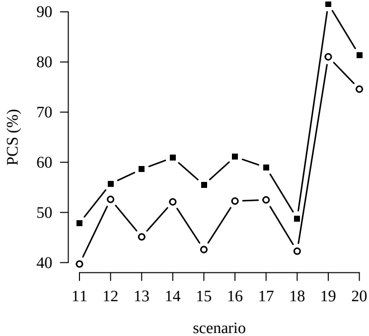
(d) PCA under \phi = 0.3
