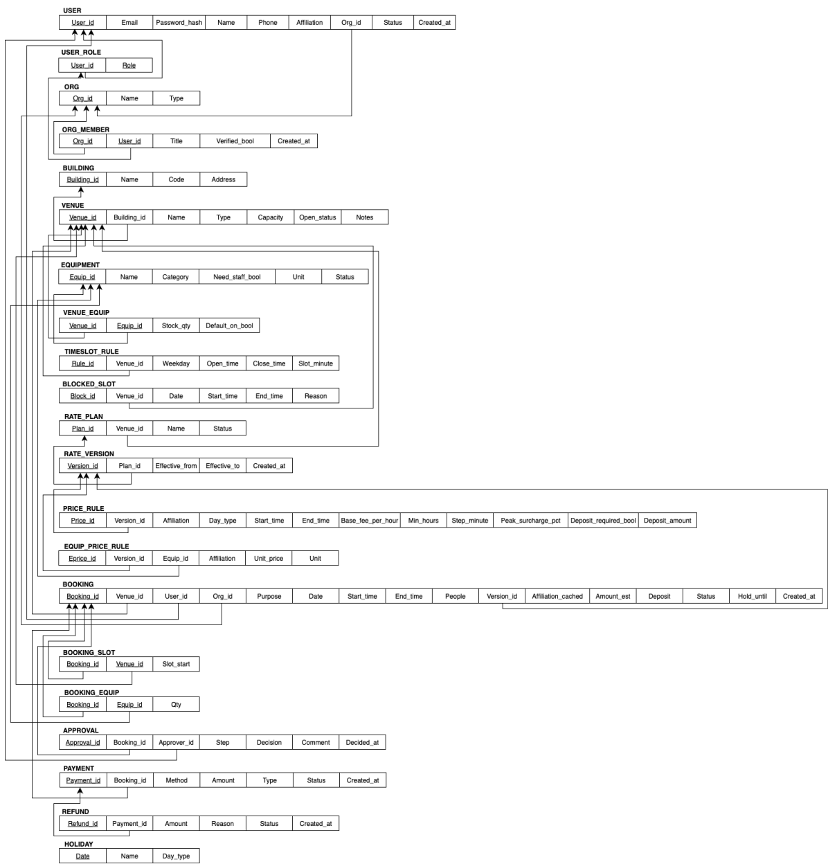
圖二：Relational Schema
