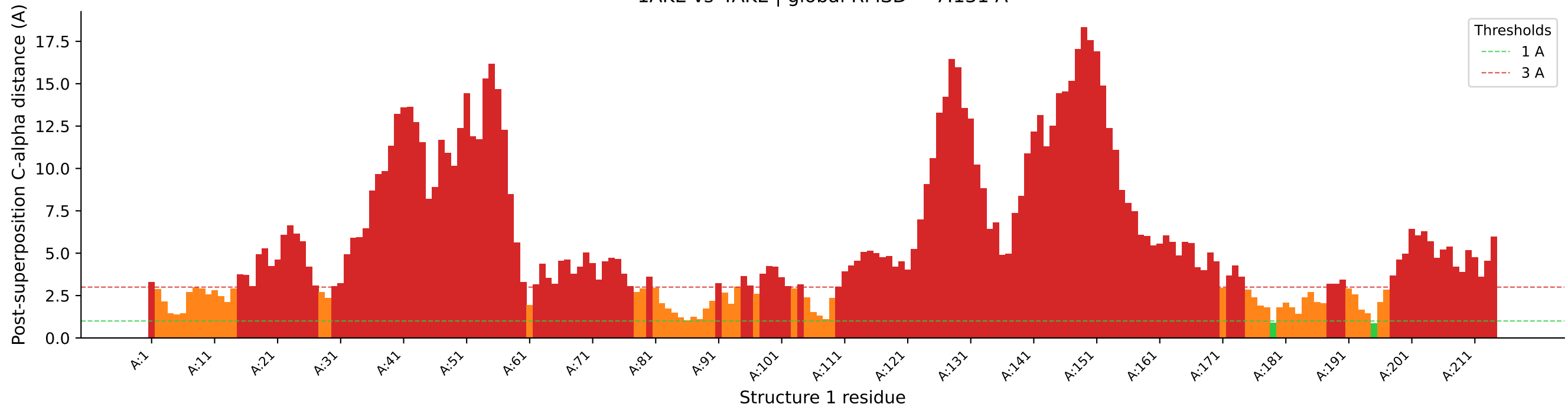
1AKE vs 4AKE | global RMSD = 7.131 Å
