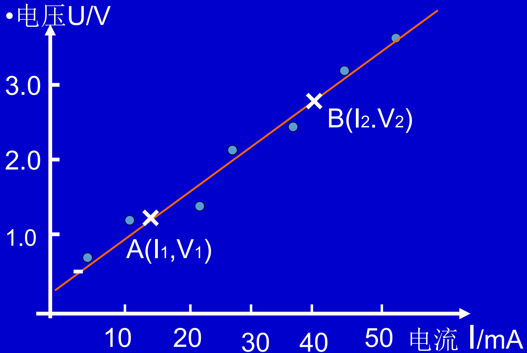
图一 交流回路中电压与电流关系
