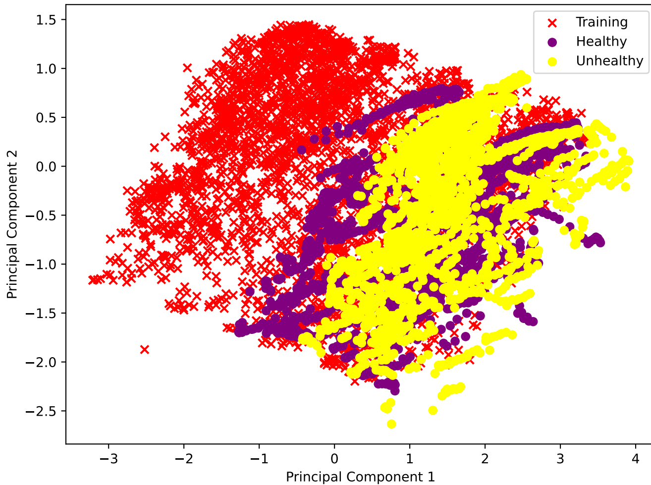
PCA Result
