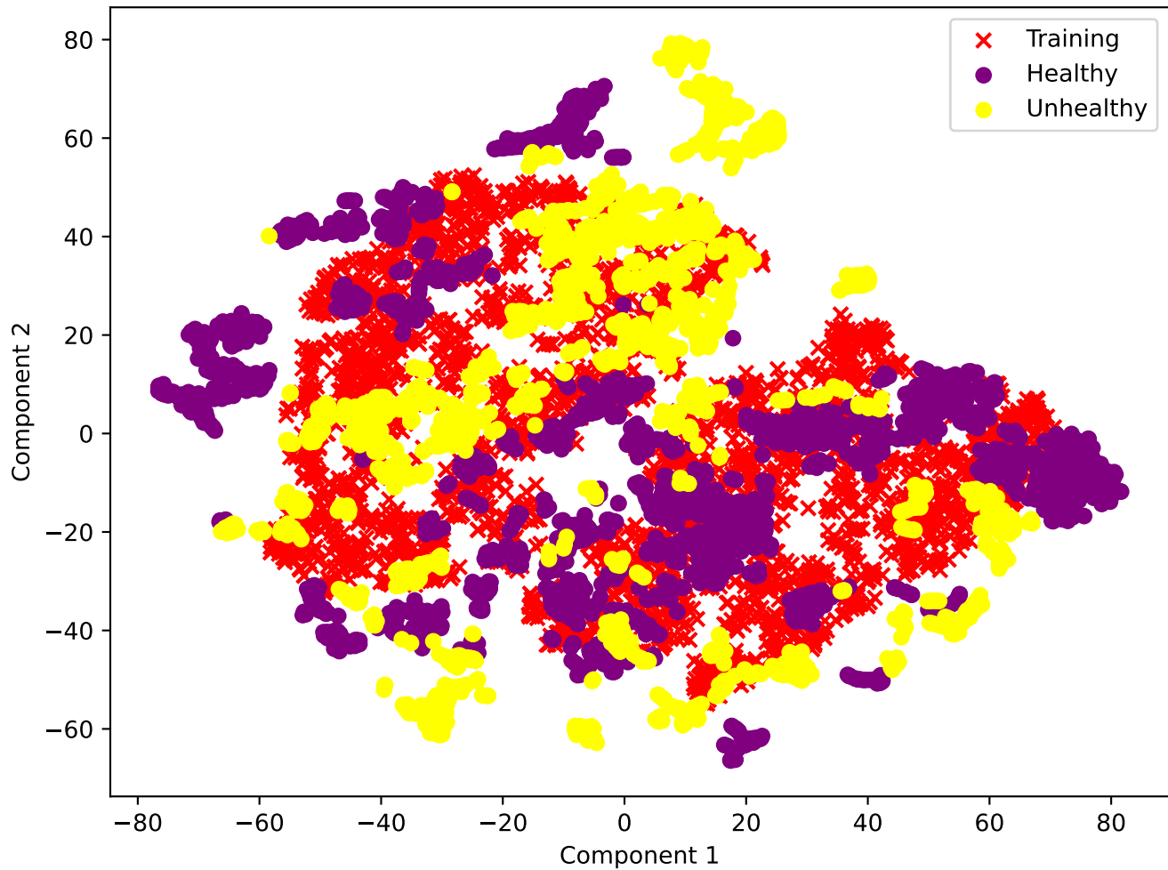
t-SNE Result
