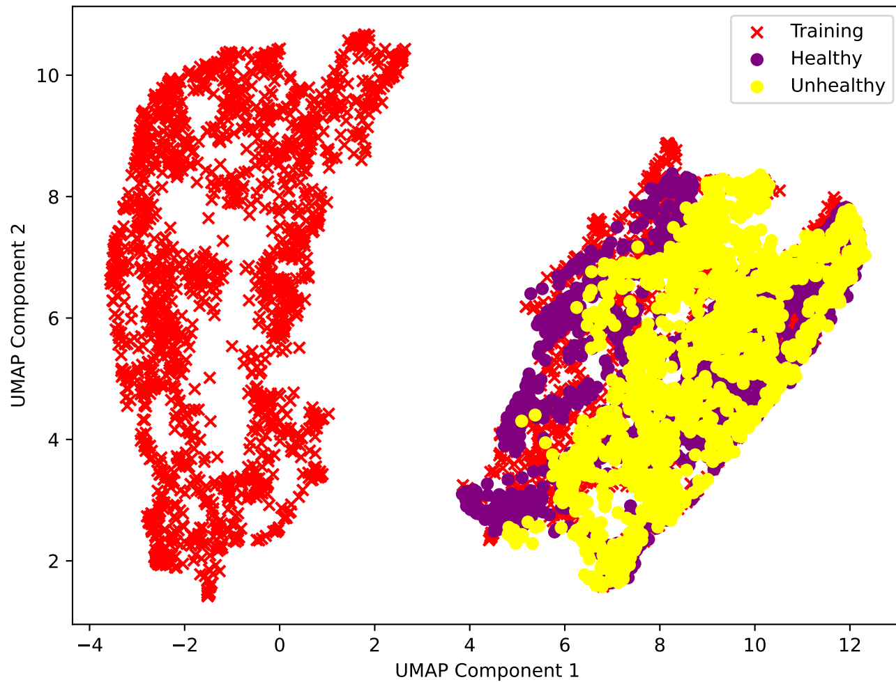
UMAP Result
