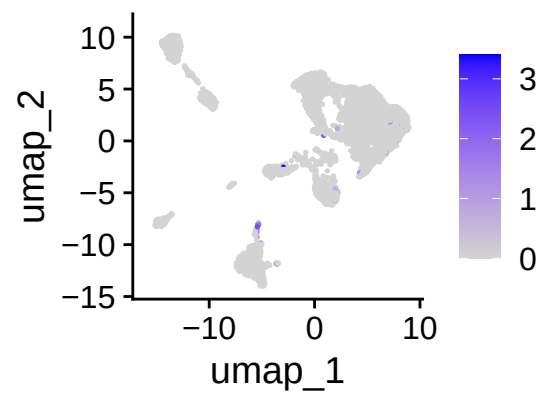
ACOT2
