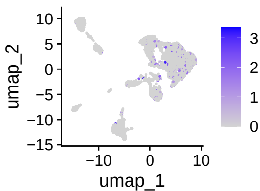
ACOX3
