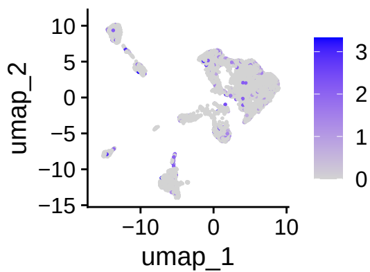
PPP6R3
