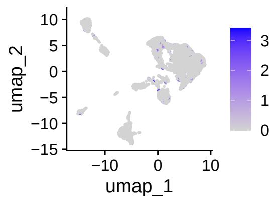
ZNF667
