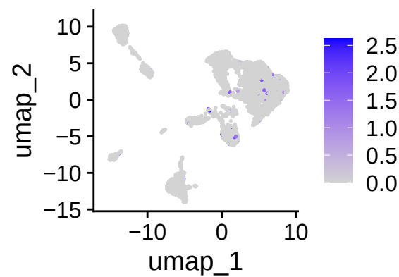
ZNF667
