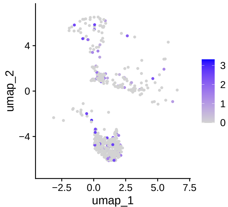
AKT2
