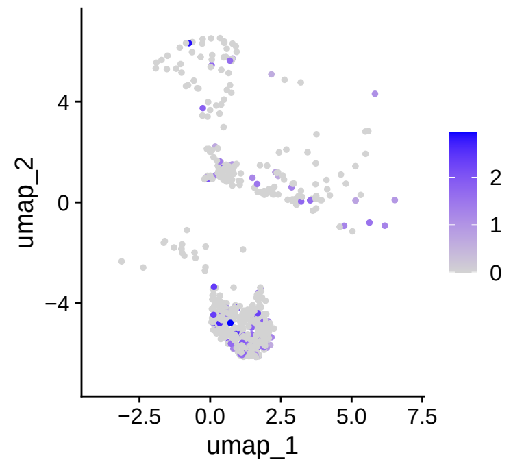
AKT3
