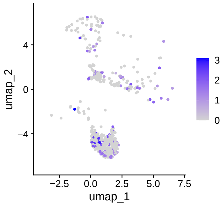
AKT1
