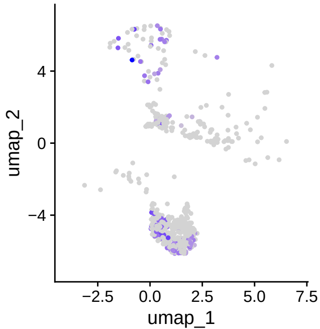
MYC
