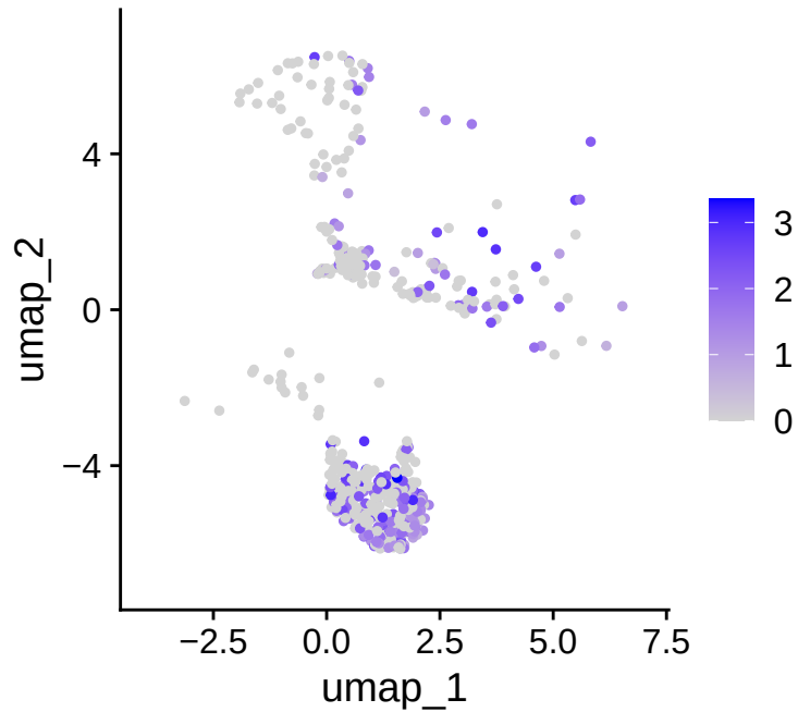
AR
