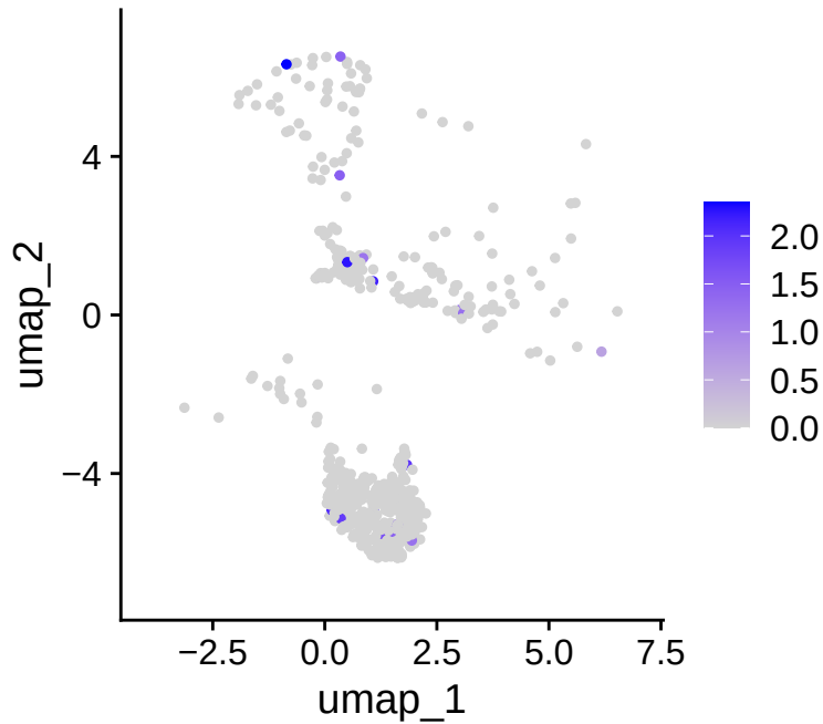
TP53
