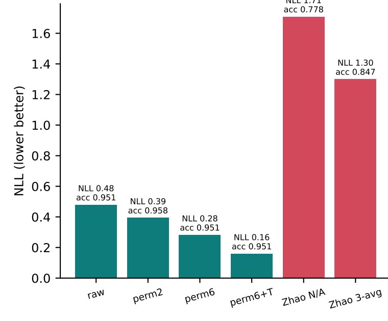
I · Calibration recipes, Gemma 4 12B Q8
