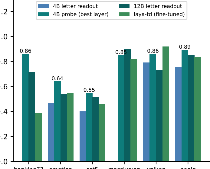
X · One probe per task, 2,000 rows
