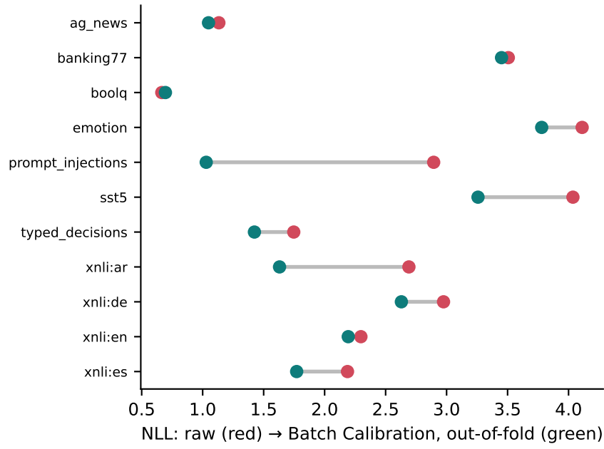
J · Batch Calibration (Zhou 2023), NLL
