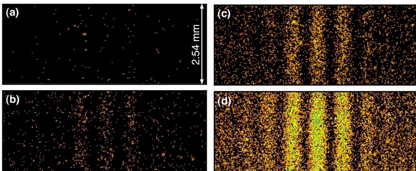
FIG. 1.9 – Observation de la construction des franges d'interférence photon par photon au moyen de la caméra CCD intensifiée. Les images (a), (b), (c) et (d) correspondent respectivement à l'accumulation de 10, 100, 500 et 2000 clichés, chacun des clichés étant associé à un temps d'ouverture de 1 s de la caméra. Le nombre de photons détecté par cliché est en moyenne égal à 10.
