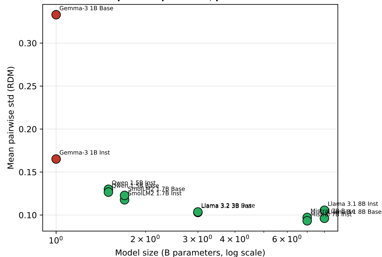
(D) RDM Std vs Size Spearman \rho = -0.891 , p = 1.0e-04
