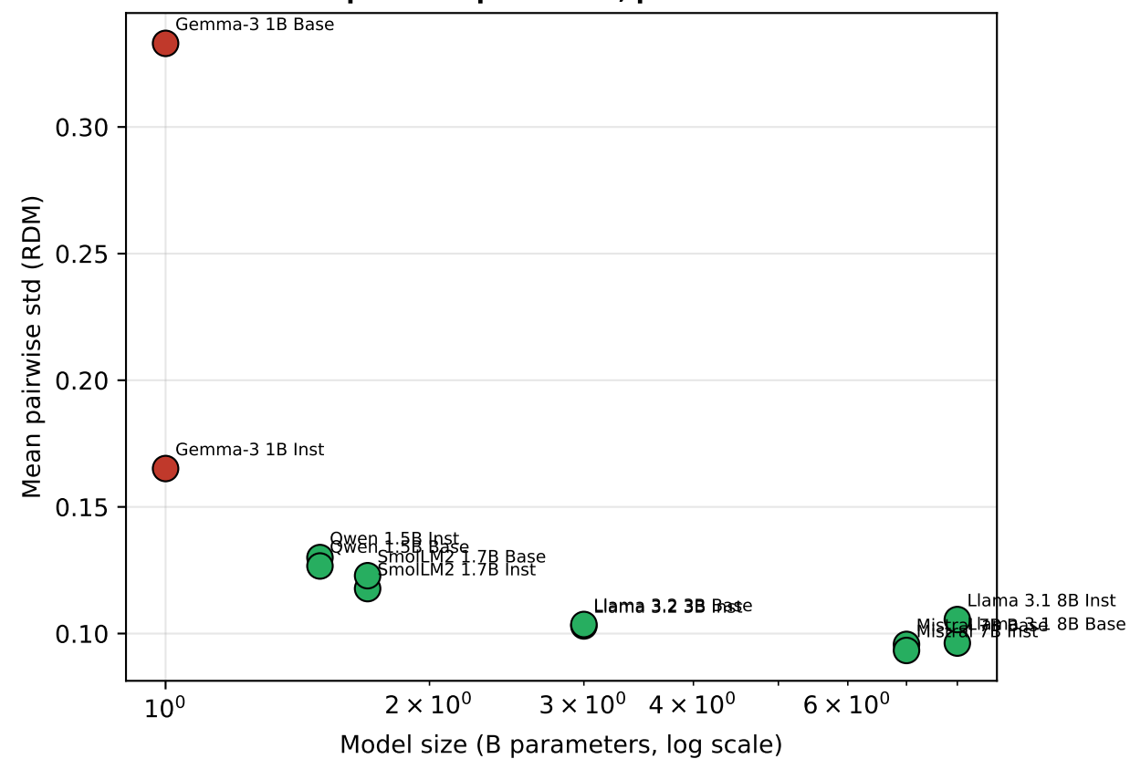
(D) RDM Std vs Size Spearman \rho = -0.876 , p = 1.8e-04
