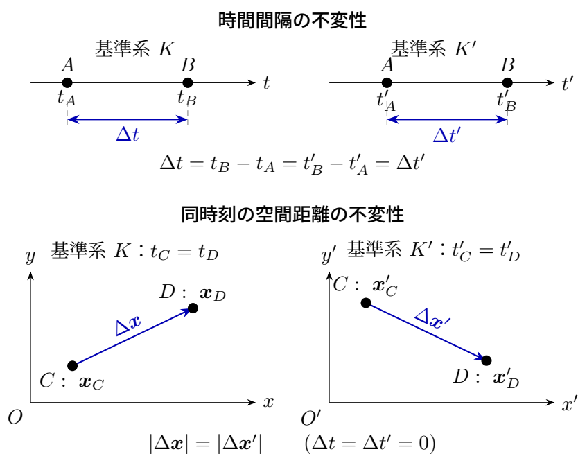
図 2 古典力学における時間間隔と同時刻の空間距離の不変性。左右は同じ事象を異なる基準系で記述したものである。空間は 2 次元で模式的に示した。
