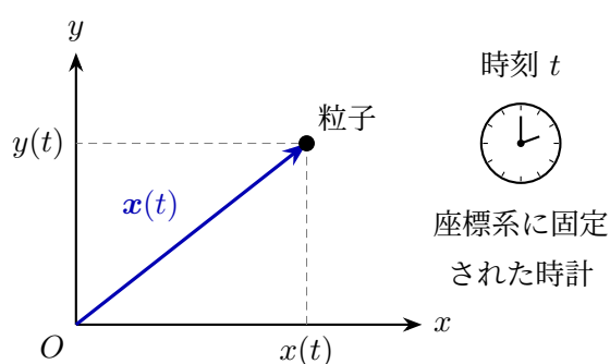
図 1 基準系を構成する空間座標系と、この系に固定された時計。空間は 2 次元で模式的に示した。
