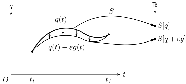
図 3 端点を固定した経路の変分と作用の変化
