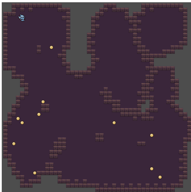
Obrázek 6: Ukázka mapy generované pomocí algoritmu Buněčných automatů (45×45)
