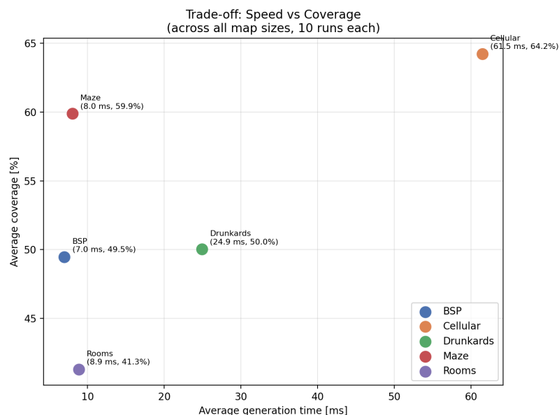
Obrázek 23: Kompromis mezi rychlostí a pokrytím (Trade-off: Speed vs Coverage)
