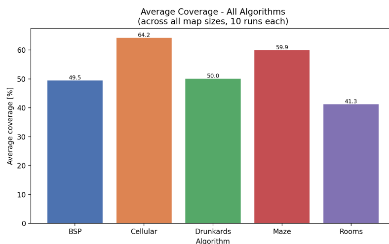
Obrázek 20: Srovnání průměrného pokrytí všech algoritmů (Average Coverage – All Algorithms)
