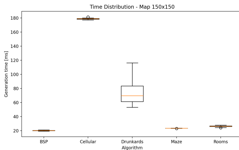
Obrázek 24: Rozptyl času generování na mapě 150 \times 150 (Time Distribution – Map 150 \times 150 )
