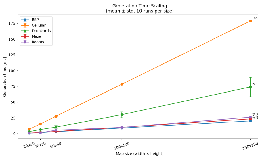
Obrázek 21: Škálování času generování s počtem buněk mapy (Generation Time Scaling)
