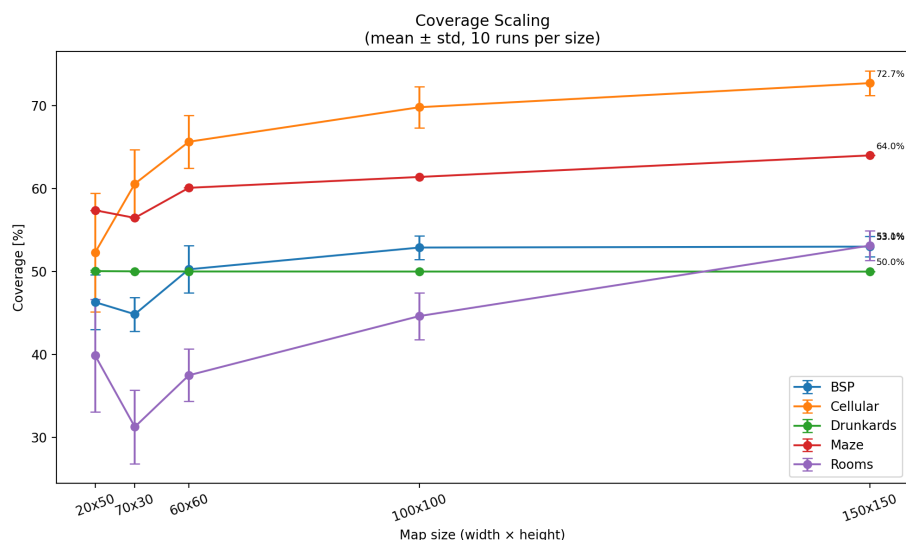
Obrázek 22: Škálování pokrytí s počtem buněk mapy (Coverage Scaling)
