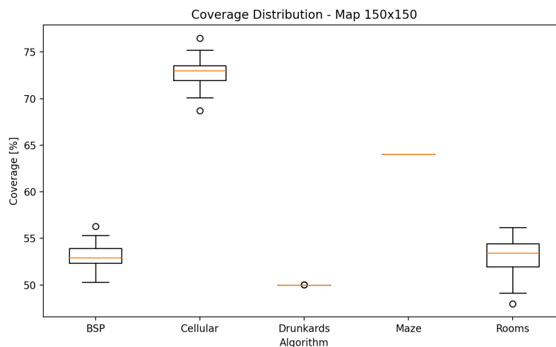
Obrázek 25: Rozptyl pokrytí na mapě 150×150 (Coverage Distribution – Map 150×150)
