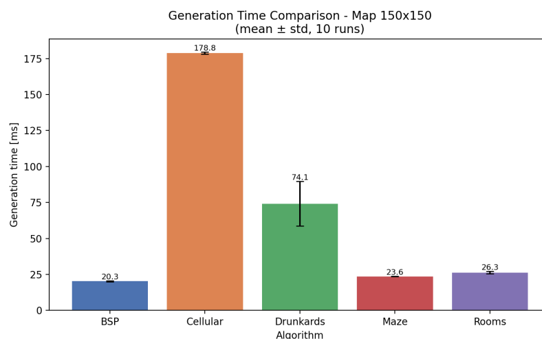
Obrázek 19: Srovnání průměrného času generování na mapě 150x150 (Average Generation Time – 150x150)
