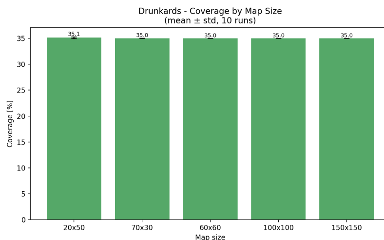
Obrázek 12: Náhodná procházka - průměrné pokrytí podle velikosti mapy (Coverage by Map Size)
