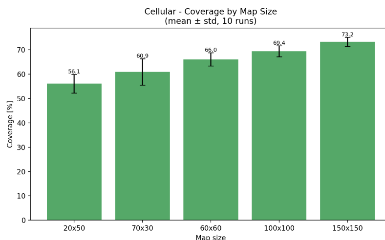
Obrázek 14: Cellular automata - průměrné pokrytí podle velikosti mapy (Coverage by Map Size)
