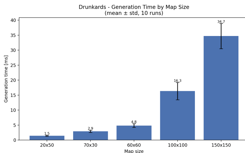
Obrázek 11: Náhodná procházka - průměrný čas generování podle velikosti mapy (Generation Time by Map Size)
