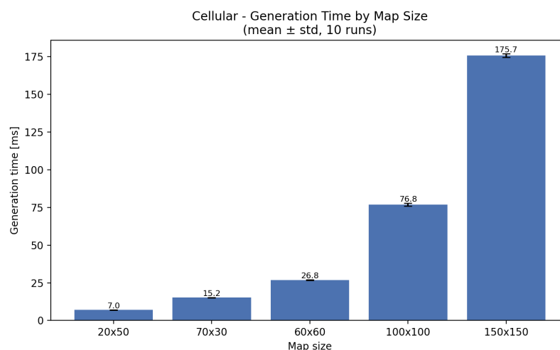
Obrázek 13: Cellular automata - průměrný čas generování podle velikosti mapy (Generation Time by Map Size)
