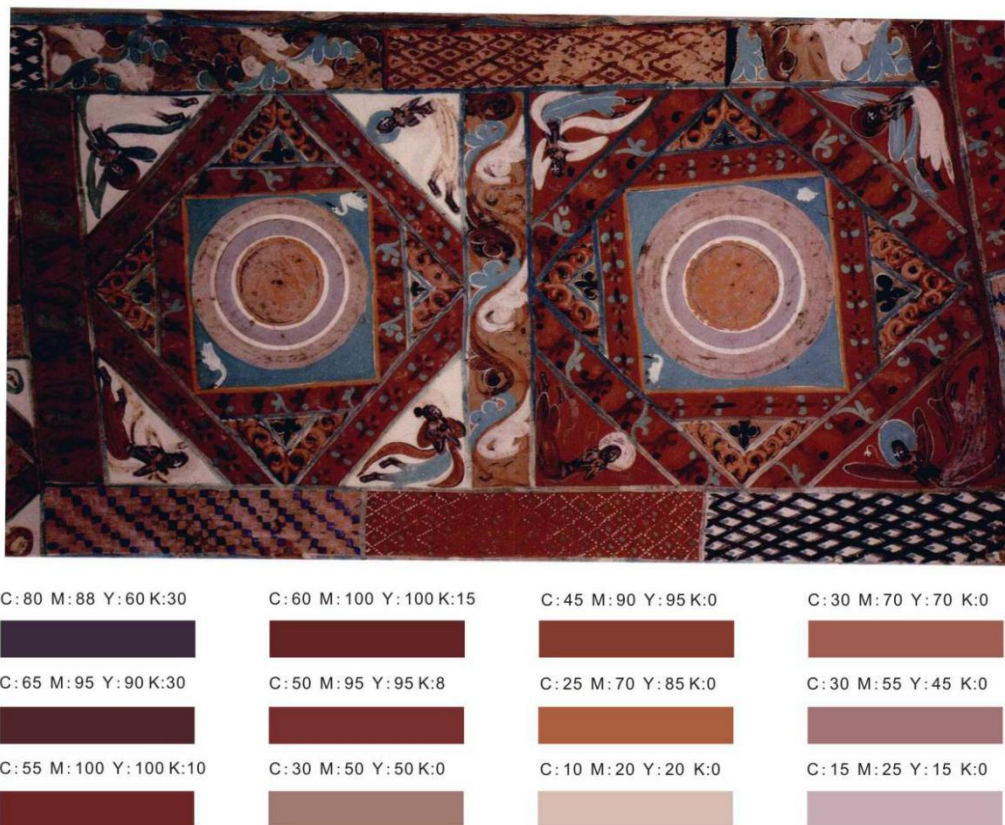
图 6-5 类似调和分析 图片来源：作者自绘
