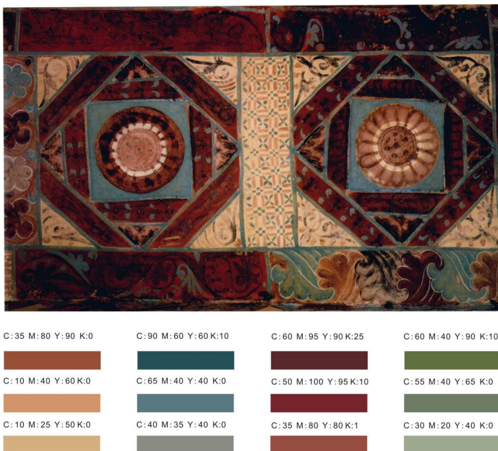
图 6-6 对比调和分析 图片来源：作者自绘
