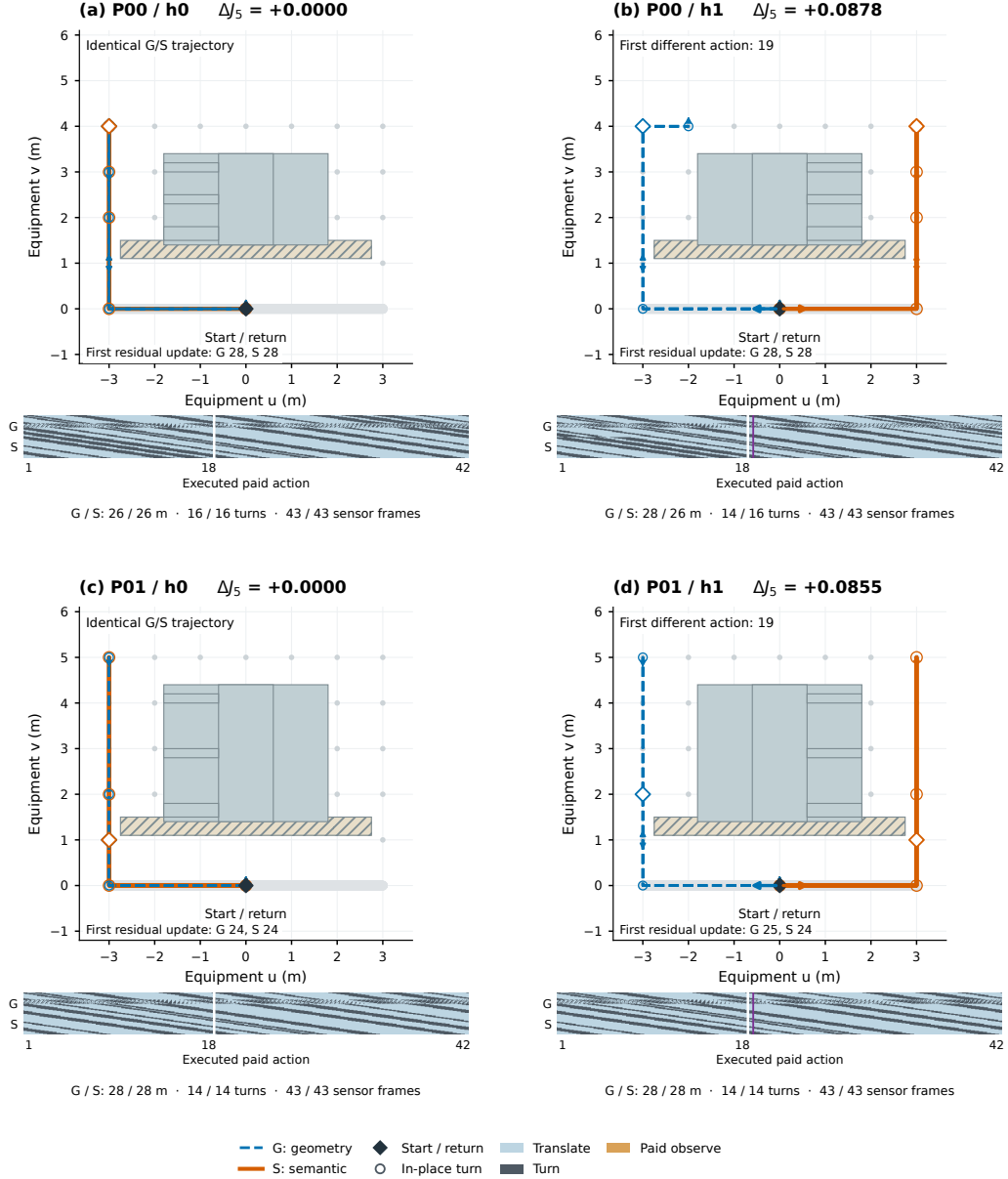
图3 四个确认条件的完整保存轨迹及逐动作带。各图采用同一米制尺度，P01 按预定义设备坐标系旋转显示；灰线表示共同 18 动作前缀，蓝虚线 G 与橙实线 S 表示后续实际路径。实心菱形为共同起终点，圆环表示原地转向位置，箭头为抽样记录的相机朝向，空心菱形为首次非零实测几何残差更新。两个 h0 条件完全同轨迹，两个 h1 条件首次执行分歧均为第 19 步。动作带保留全部平移及转向，避免重合路径隐藏观察代价。背景完整几何仅用于离线解释。
