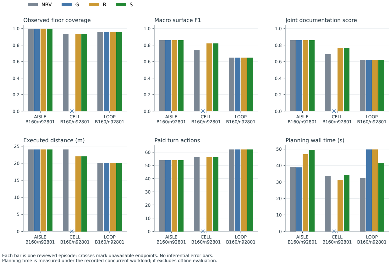
图 15 原流程合格终点的覆盖、全实例宏平均 F1、联合分数及实际成本。每根柱对应一条任务，无推断性误差条；叉号表示该快照未纳入的原评价失败项，不表示零质量或零路程。规划耗时排除离线表面评价，受到当时并发负载影响，不据此进行严格硬件归一化速度排名。
