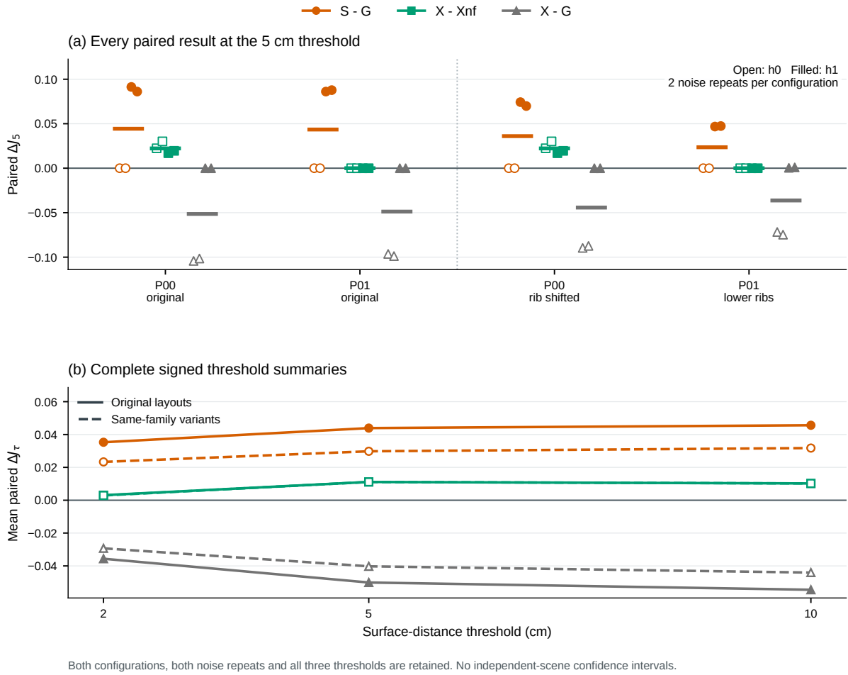
图 12 42 步下原布局 and 同族结构变体的完整配对差及 2/5/10 cm 敏感性。类别、整体纠错和错误类别三个对比均按相同场景、构型、种子配对；小点显示重复条件，均值不附独立场景置信区间。两个变体属于已声明设施族内的几何扰动。
