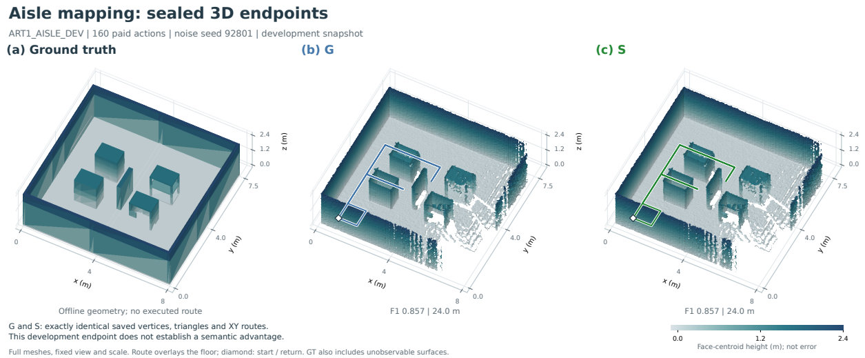
图 16 AISLE 完整真值与保存的 G、S 终点 TSDF，共享正交视角、世界范围及米制尺度。每份预测的全部 205,566 个三角面参与显示，无抽稀、补洞或模板补面；XY 路线投影到地面并覆盖遮挡显示，菱形表示起点与返航位置。颜色表示三角面中心高度和几何光照，不表示误差。G/S 网格及路径相同。GT 包含不可观测表面，而指标使用固定可观测参考。
