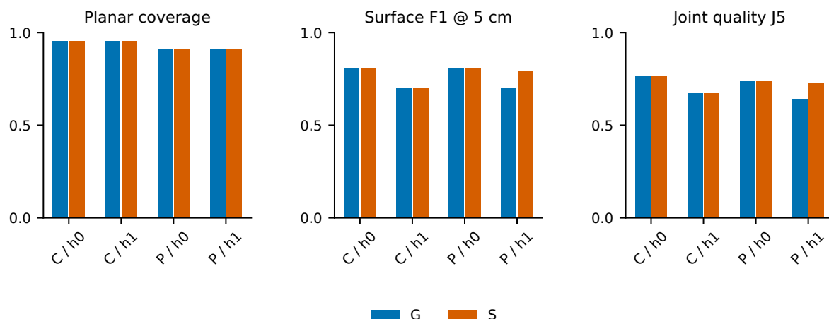
图 25 四个配对条件的覆盖、表面 F1 及联合指标。C/P 分别表示侧柱和后隔台布局。全部持平与正差均保留，纵轴统一为 0—1；不附加跨独立布局的显著性结论。
