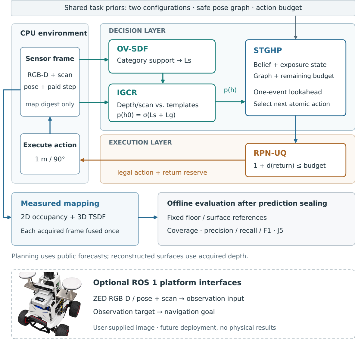
图 1 平台接口、四模块 CPU 虚拟验证与独立重建评价。OV-SDF 和 IGCR 共同更新构型信念，STGHP 选出下一原子动作，经 RPN-UQ 检查后执行并获取新观测。公开模板支持信念与规划，TSDF 仅融合实测深度，真值仅用于输出封存后的评价。小车为未经内容修改的用户供图，用于后续 ROS 1 接口说明；流程框线由程序绘制为矢量图，性能结论来自 CPU 仿真。
