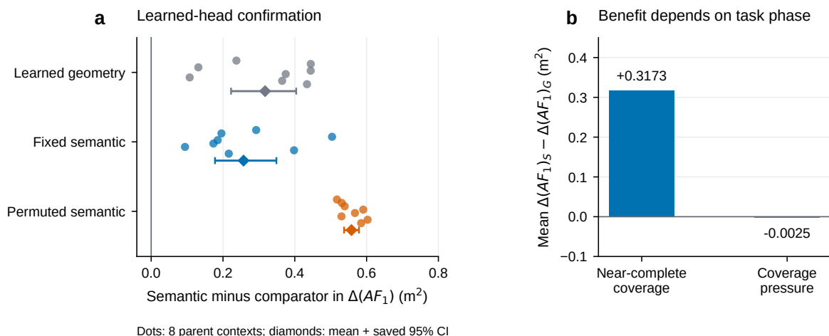
图 9 学习型收益头的独立证据与失效边界。(a) 散点为 8 个父上下文的配对平均差，菱形及横线为均值与原保存组级 bootstrap 区间；确定性纵向错位仅便于辨认。(b) 语义减同容量几何的面积联合增量差：接近覆盖完成时为正，覆盖压力层接近零且略负。两层独立成组，不与 V35/V36 的归一化 J_5 混合。
