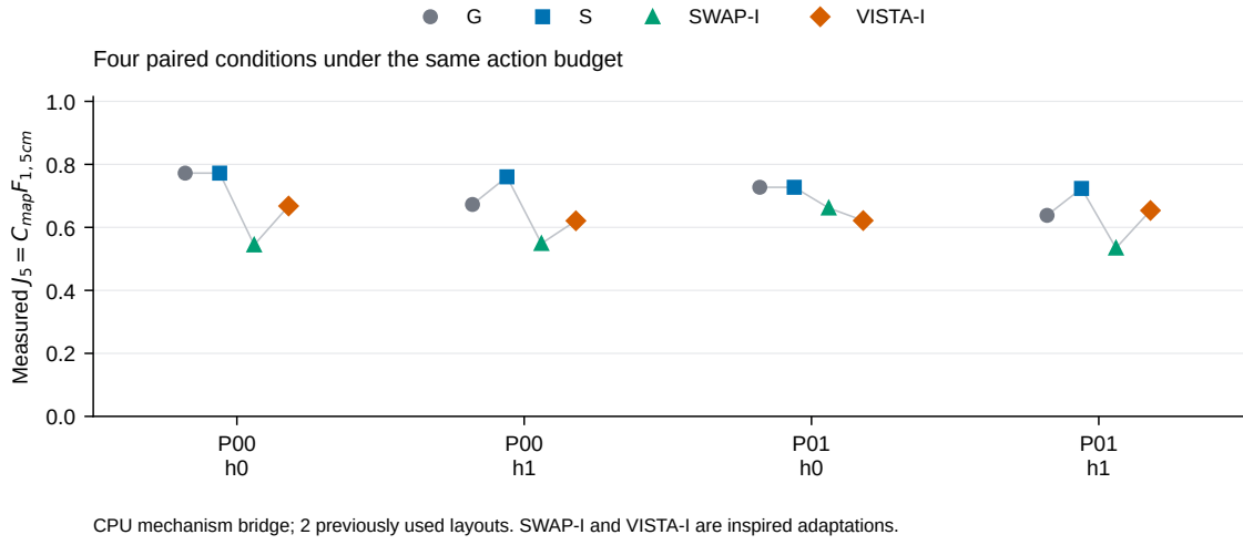
图 6 四个已知布局/构型条件中的共同 CPU 联合终点。点为完整执行结果，灰线仅连接同一条件，不表示时间演化或置信区间；独立复现未重复画作样本。
