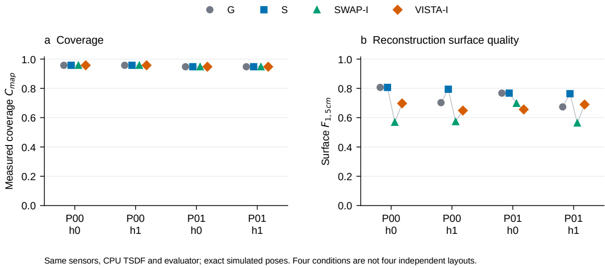
图 7 共同 CPU 比较的二维覆盖与三维表面质量分解。相同条件内覆盖相等，联合分数差来自 F1；绝对分数轴从零开始。
