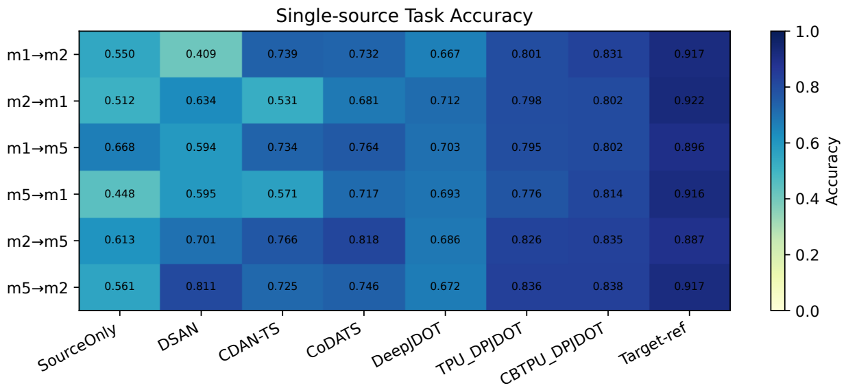
图 6-2 单源跨工况逐任务目标域准确率热力图
