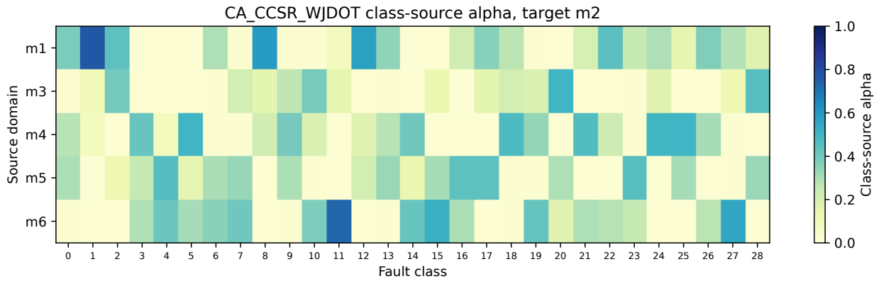
图 6-8 五源任务 \{m_1, m_3, m_4, m_5, m_6\} \rightarrow m_2 中 CA_CCSR_WJDOT 的源域–类别权重热力图
