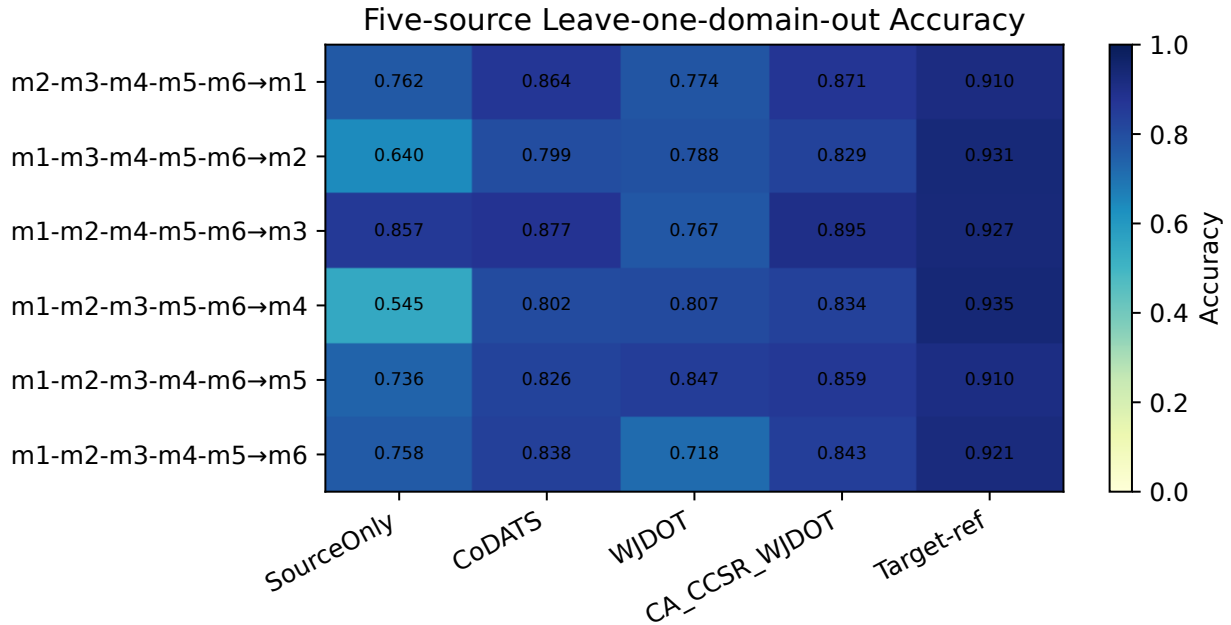
图 6-5 五源留一域逐目标生产模式准确率热力图
