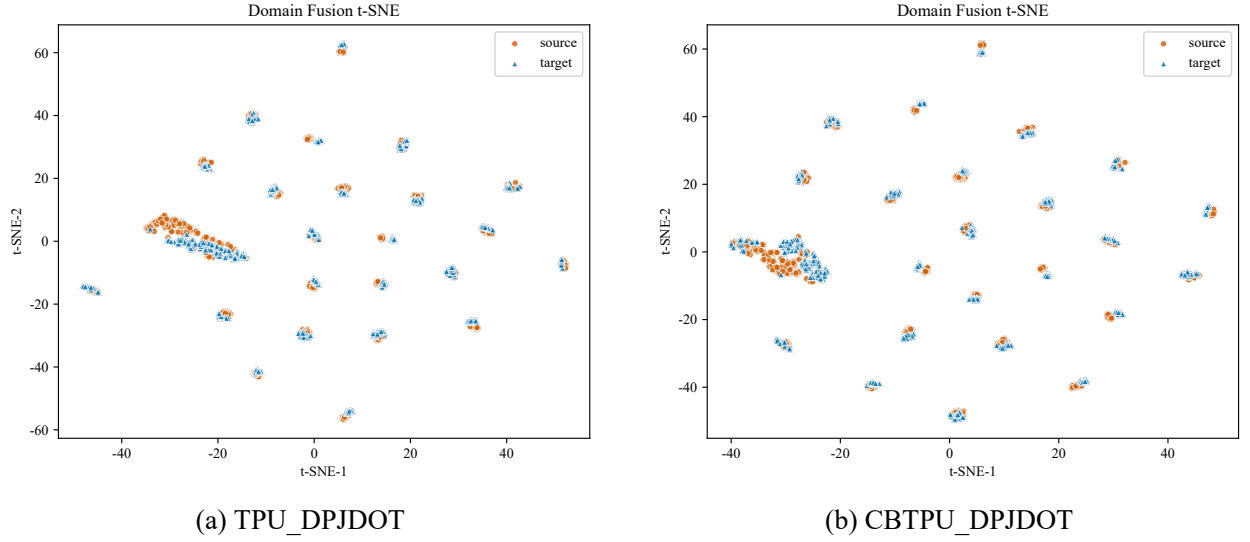
图 6-6 单源任务 m_5 \rightarrow m_2 中 TPU_DPJDOT 和 CBTPU_DPJDOT 的域 t-SNE 对比
