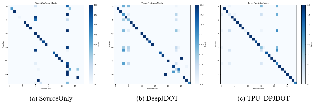
图 6-2 单源任务 m_5 \rightarrow m_2 中 SourceOnly、DeepJDOT 和 TPU_DPJDOT 的目标域混淆矩阵对比
