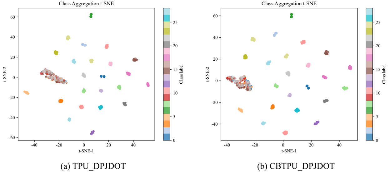
图 6-7 单源任务 m_5 \rightarrow m_2 中 TPU_DPJDOT 和 CBTPU_DPJDOT 的类 t-SNE 对比
