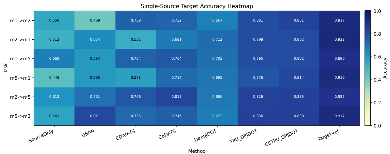
图 6-11 单源跨工况 8 种方法逐任务目标域准确率热力图
