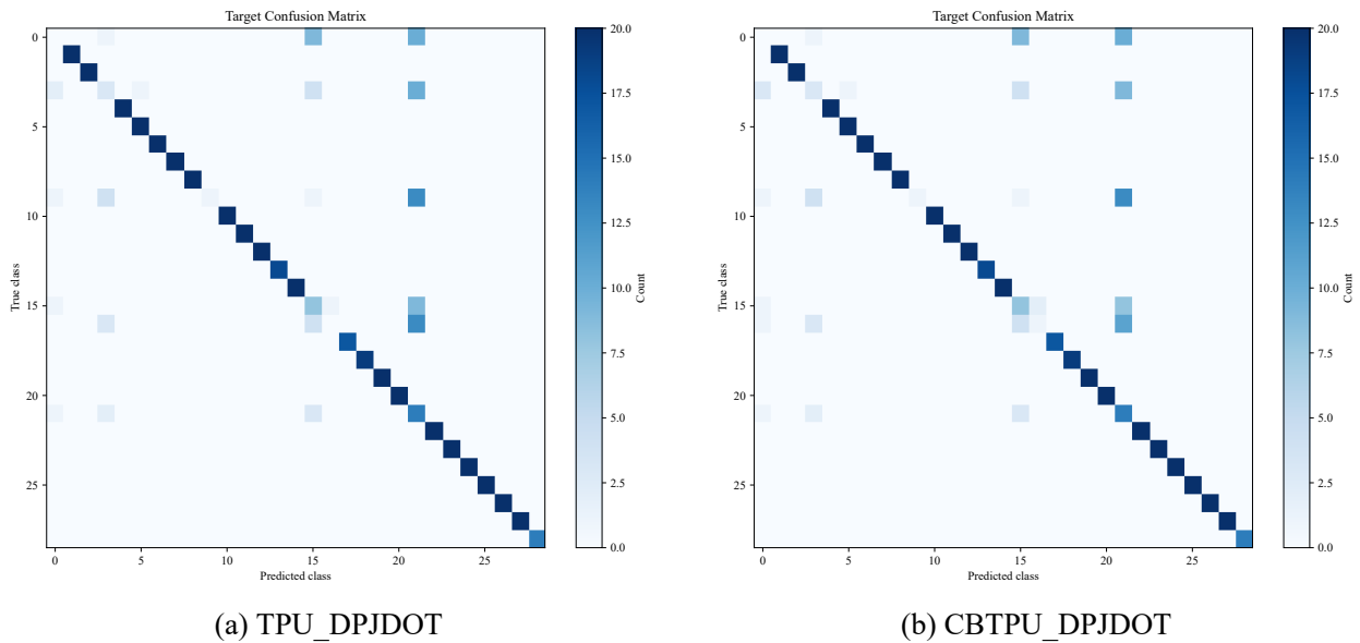
图 6-5 单源任务 m_5 \rightarrow m_2 中 TPU_DPJDOT 和 CBTPU_DPJDOT 的目标域混淆矩阵对比
