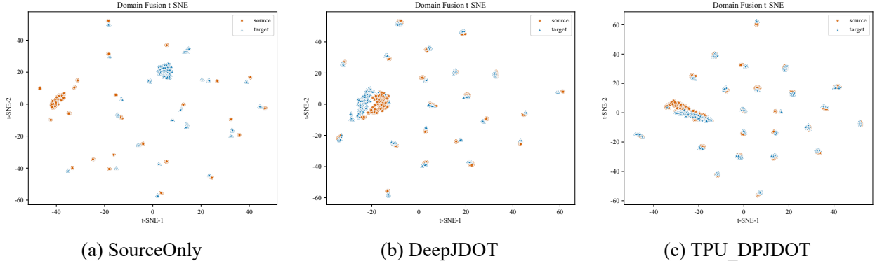
图 6-3 单源任务 m_5 \rightarrow m_2 中 SourceOnly、DeepJDOT 和 TPU_DPJDOT 的域 t-SNE 对比
