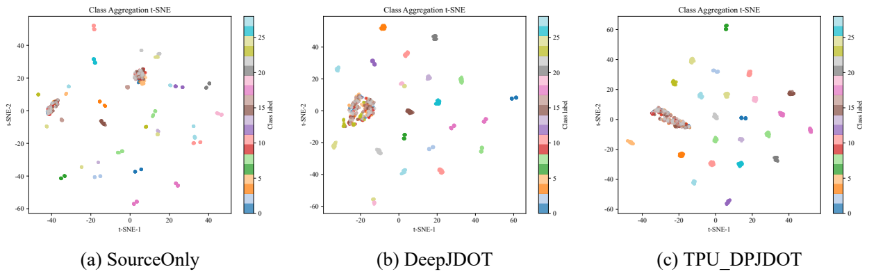
图 6-4 单源任务 m_5 \rightarrow m_2 中 SourceOnly、DeepJDOT 和 TPU_DPJDOT 的类 t-SNE 对比
