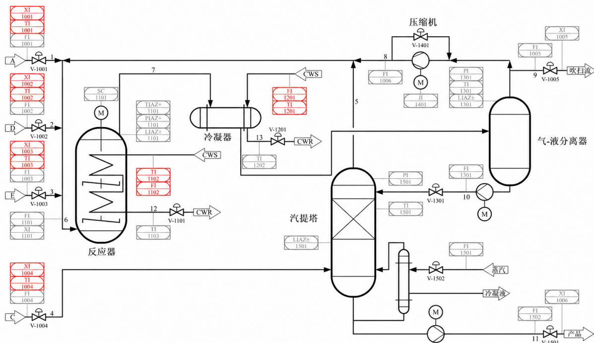
图 6-1 田纳西伊斯曼工艺流程示意图
