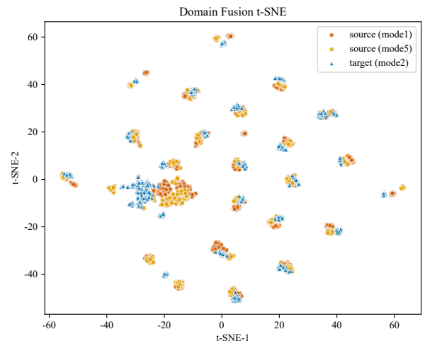
(d) CA-CCSR-WJDOT
