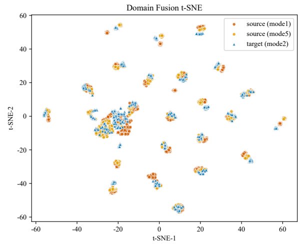
(b) CoDATS
