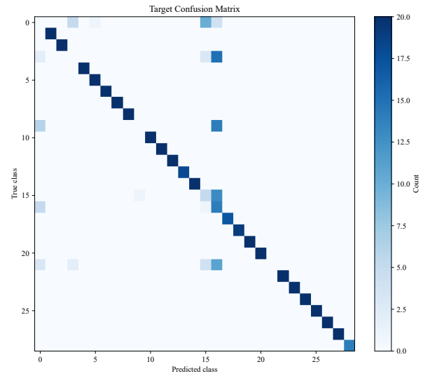
(d) CBTPU-DJDOT
