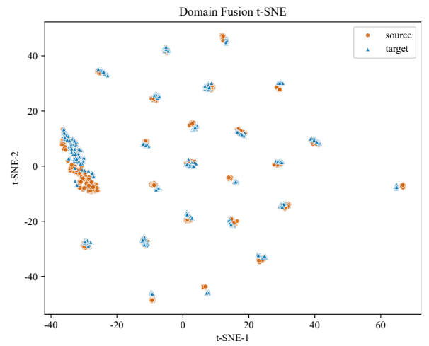
(d) CBTPU-DJDOT
