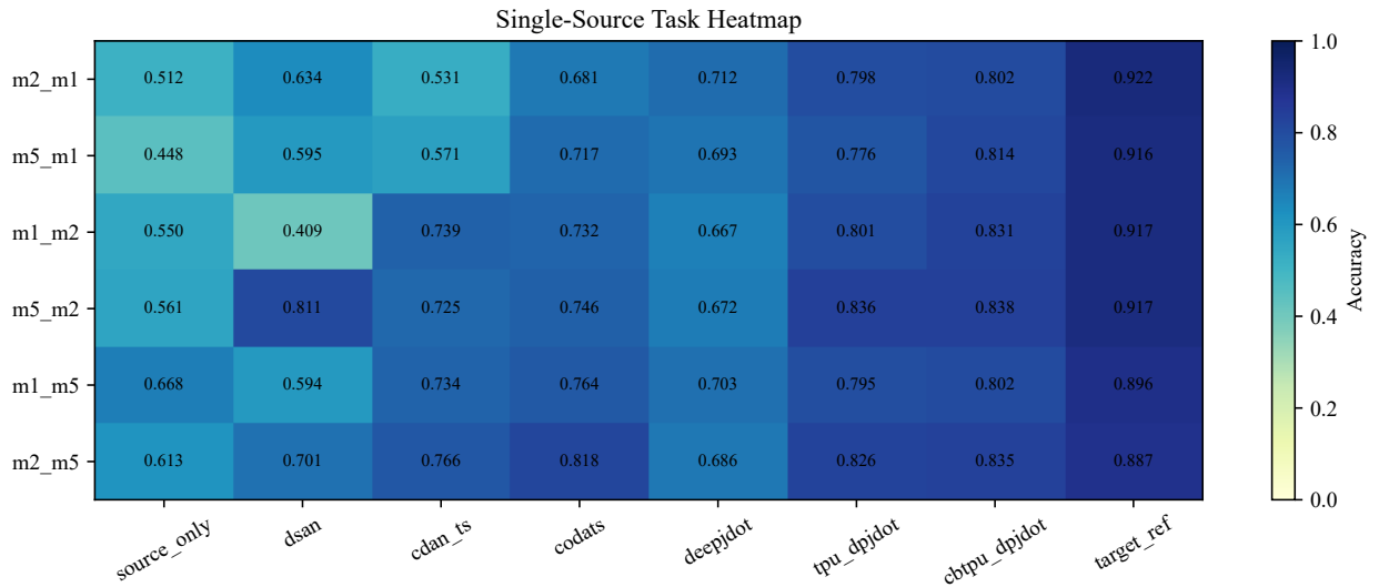
图 6-3 单源跨工况完整基线逐任务目标域准确率热力图
