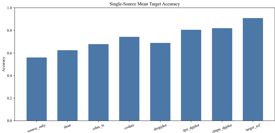
图 6-2 单源跨工况完整基线平均目标域准确率柱状图
