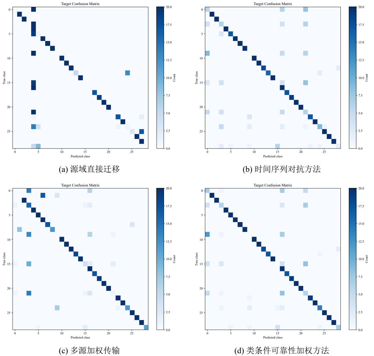
图 6-8 五源任务 \{m_1, m_3, m_4, m_5, m_6\} \rightarrow m_2 中代表方法的目标域混淆矩阵
