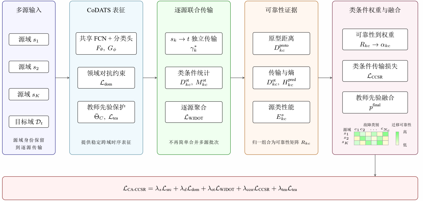
图 3: 类条件源域可靠性加权多源方法架构示意
