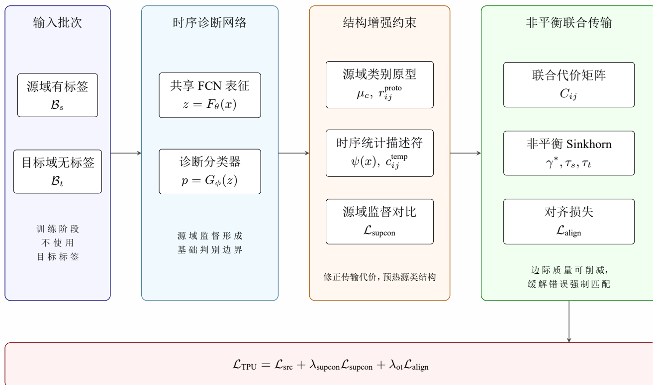
图 1: 时序原型非平衡联合分布对齐方法架构示意
