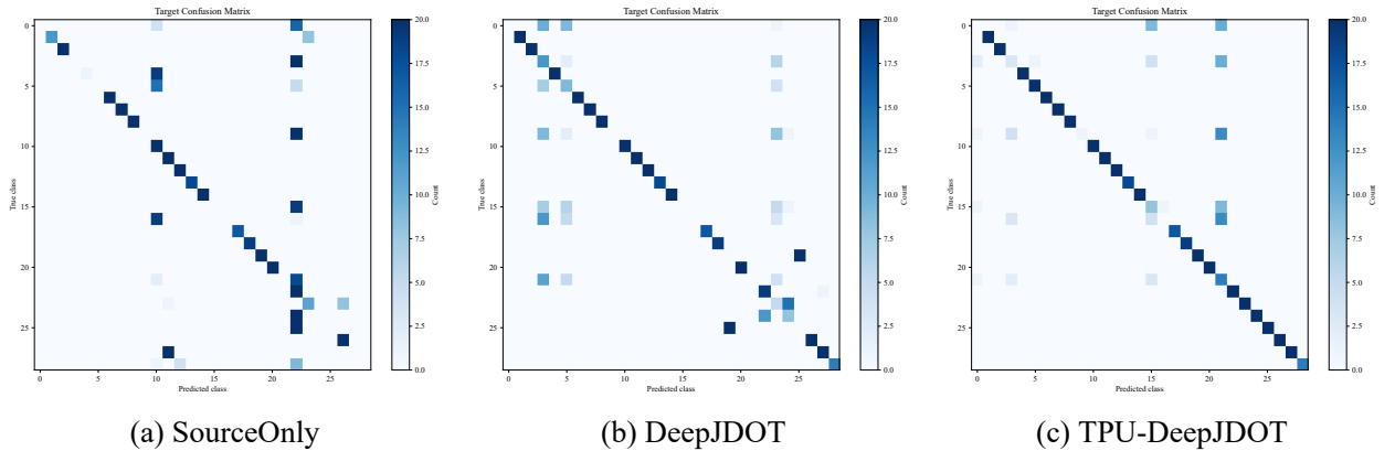
图 6-2 单源任务 m_5 \rightarrow m_2 中 SourceOnly、DeepJDOT 和 TPU-DeepJDOT 的目标域混淆矩阵对比
